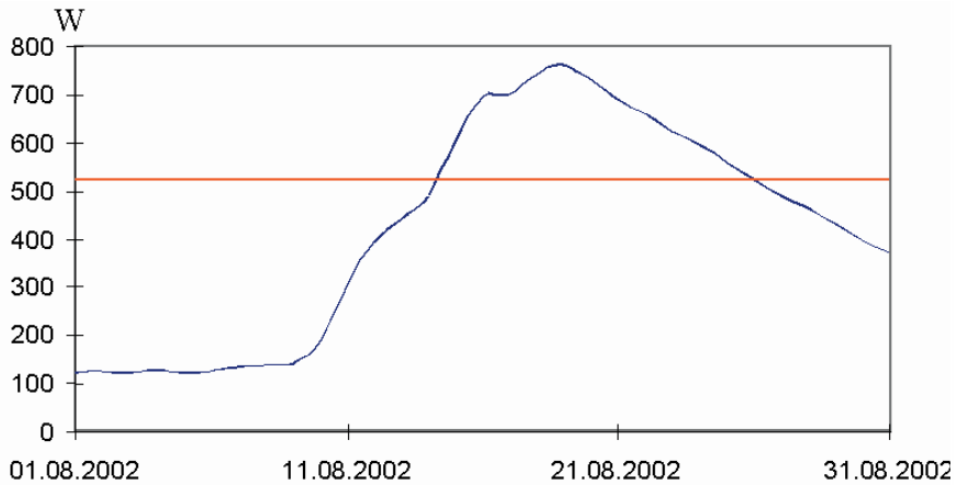
Abb. 9 Verlauf des Sommerhochwassers 2002 am Pegel Aken (Quelle: WSA Dresden).
