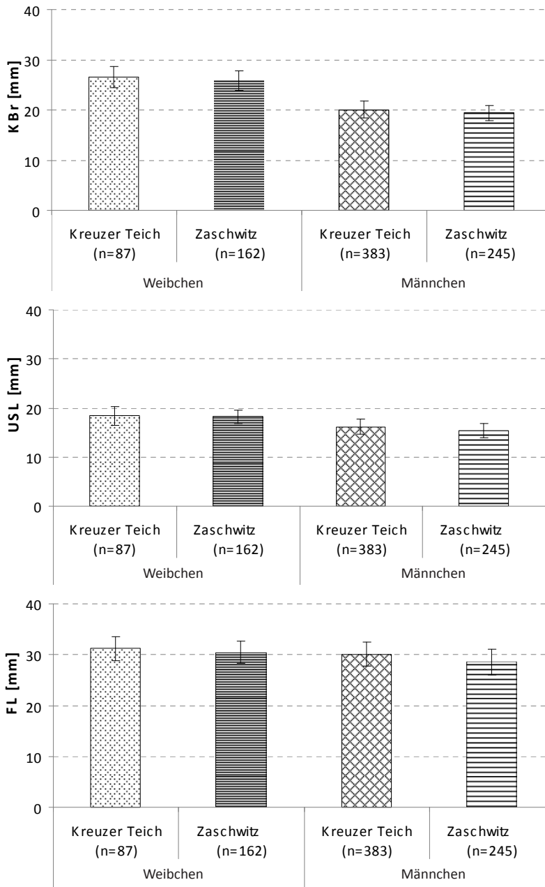
Abb. 11 Vergleich der Individuen beider Populationen hinsichtlich ihrer Kopf­breite (KBr in mm; Grafik oben), Unterschenkel­länge (USL in mm; Grafik Mitte) und Fußlänge (FL in mm; Grafik unten). Dargestellt sind die Mittelwerte und die jeweilige Standardabweichung.
