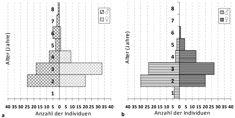
Abb. 7 Alterspyramiden für die Erdkröten der Untersuchungsgebiete Kreuzer Teich (a) und Zасschwitz (b). Säulen in (a) und (b) links: Männchen. Säulen rechts: Weibchen.
