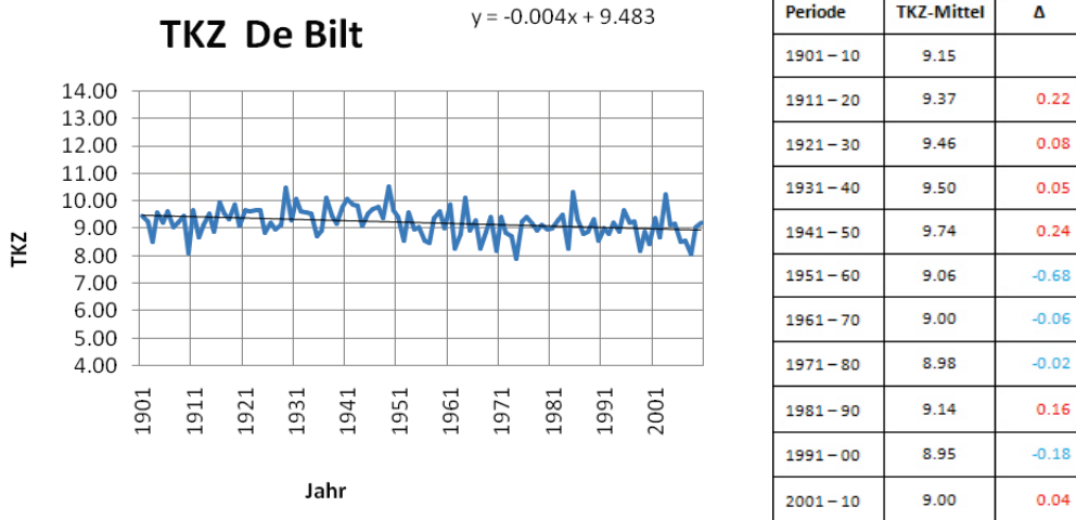
Abb. 2 Zeitlicher Verlauf der jährlichen TKZ sowie Pentadenmittel auf dem Hohenpeißenberg.
