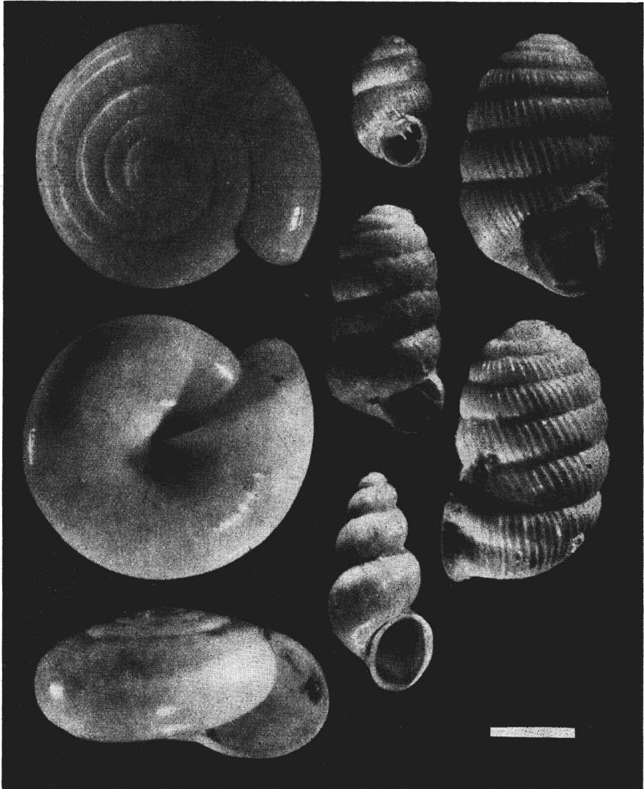
Tafel 1. Kleine Schnecken aus hochinterglazialem Travertin:
