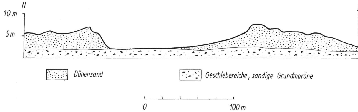
Profil 1. Querprofil durch die nördliche Parabeldüne bei Seppin
