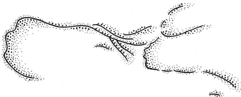
Karte 1. Dünen in der östlichen Litzinger Heide
