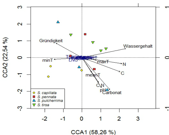
Abb. 8 Kanonische Korrespondenzanalyse (CCA). Einfluss von abiotischen Faktoren auf den CWM der funktionellen Merkmale für die verschiedenen Stipa -Rasen im Raum der ersten und zweiten Hauptkomponente. Umweltvariablen sind als Vektorpfeile dargestellt (meanT (durchschnittliche Temperatur), maxT (maximale Temperatur), minT (minimale Temperatur), Gründigkeit, Wassergehalt, pH-Wert, N-Gehalt, C-Gehalt, C.N (C/N-Verhältnis), Carbonatgehalt). Funktionelle Merkmale (Wuchshöhe, Blatttrockenmasse, Blattfläche, LDMC, SLA, LNC, LCC, C.N (C/N-Verhältnis)) sind als Zentroide dargestellt (blaue Schrift). Symbole und Farben entsprechen den Plots (Datensatz über 13 Plots) der jeweiligen Stipa -Rasen. Die Anteile erklärter Variabilität sind an den Achsen angegeben. Das Ergebnis ist für das Gesamtmodell nicht signifikant (999 Permutationen, p = 0,4 ).
