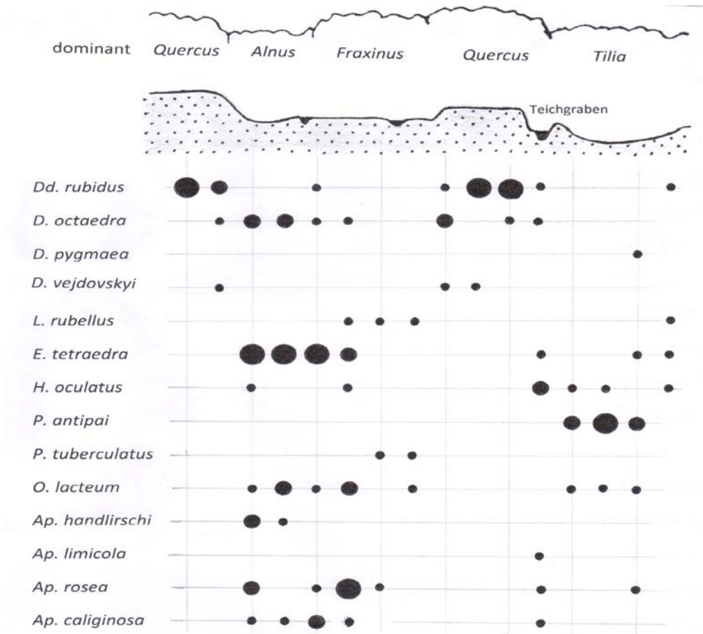
Abb. 2 Regenwurmfauna in einem Geländeschnitt durch den nordwestlichen Teil des Leinawaldes: • 1-3, • 4-10 und • >10 adulte Individuen auf 0,25 m² untersuchter Fläche.
