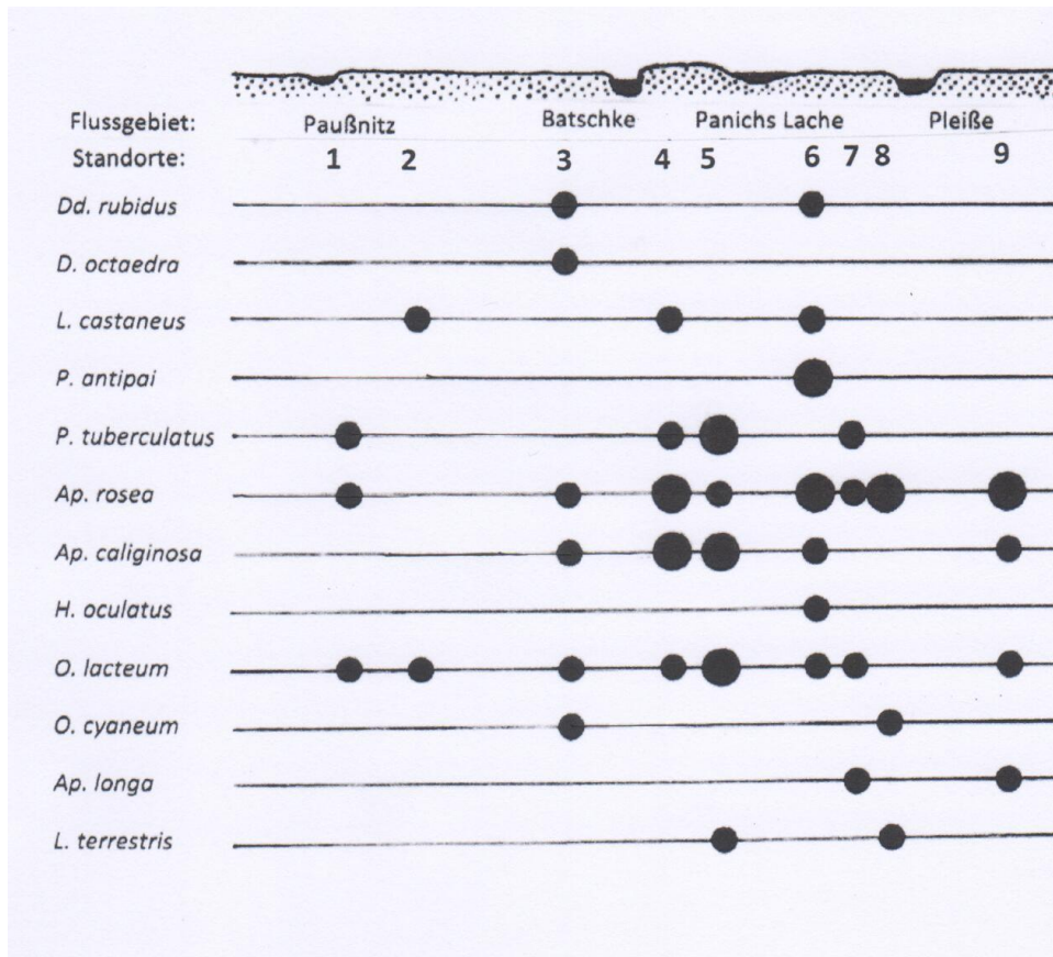
Abb. 3 Querschnitt durch die Regenwurmfauna des Südlichen Leipziger Elster-Pleisse-Auenwalds. – Individuendichte der Adulti: • 1 bis 5 Ind./ 0,25 m²; • >5 Ind./ 0,25 m².
