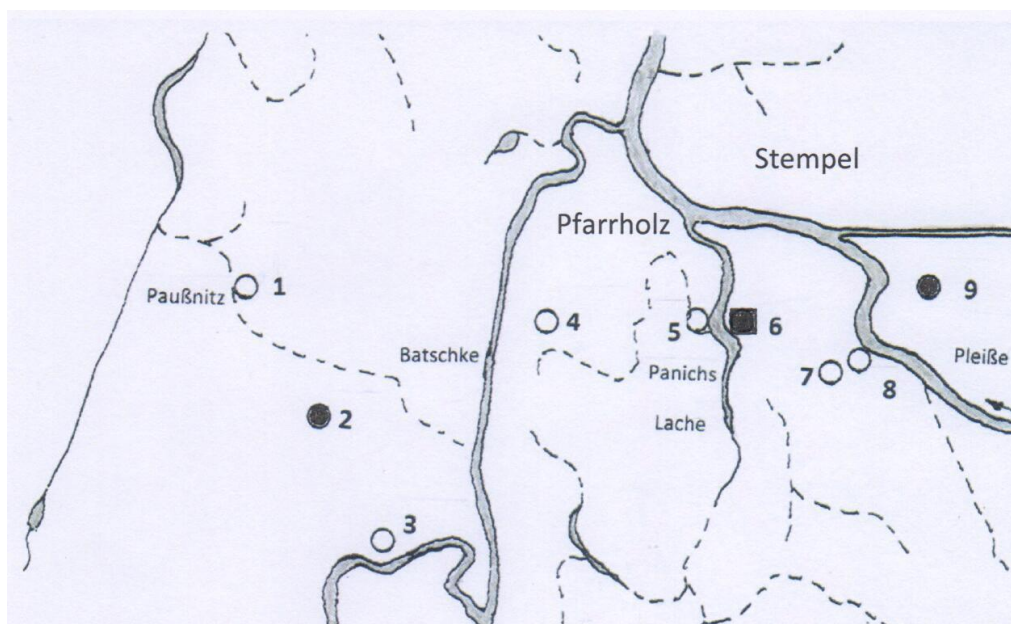
Abb. 2 Ausgewählte Bodenstandorte Nr. 1 bis 9 im Querschnitt des Südlichen Elster-Pleiße-Auenwalds. Charakter des Standorts: ○ flussnah, mit Fluvisoliment; ● flussfern, ohne Fluvisoliment; ■ stark hydromorph.
