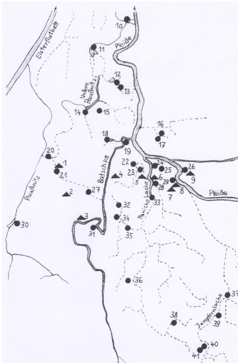
Abb. 1 Übersicht über die 41 untersuchten Bodenstandorte in der Südlichen Elster-Pleiße-Aue in Leipzig. ▲ Bodenstandorte 1-9 vorgestellt in Abb. 2 und 3.
