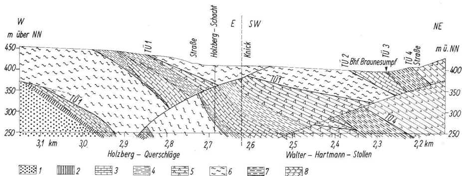
Abb. 3. Vereinfachter Schnitt vom Holzberglager der Grube Braunesumpf über das Nordende der Leibfahrscholle und die Kulmscholle vom Forstort Öhrental bis in die Wissenbacher Schiefer
