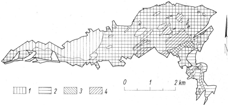
Abb. 2. Versuch einer Alterseinstufung der am Michaelsteiner „Hauptquarzit“-Zug und den Hüttenröder Schichten beteiligten Gesteine Zur Topographie vgl. Abb. 1; 1: Unterdevon; 2: Mitteldevon; 3: Oberdevon; 4: Unterkarbon
