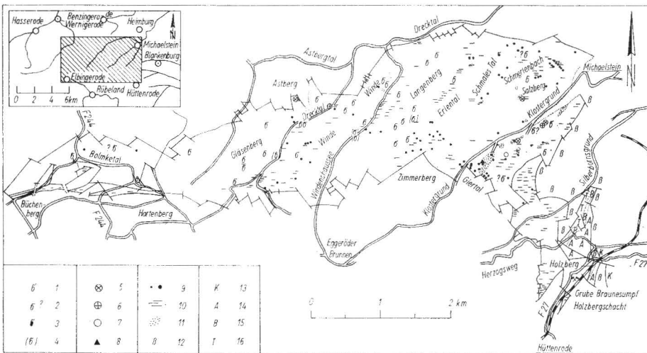
Abb. 1. Gebiet des Michaelsteiner „Hauptquarzit“-Zuges und der Hüttenröder Schichten 1: Fossilfundpunkt mit Oberemsfauna; 2: desgl., Lage fraglich; 3: desgl., fragliches Oberems; 4: Fossilfundpunkt mit vermutlicher Mitteldevonfauna in kalkigen Schiefen; 5: Flinzkalk mit Eifel fauna (bis unt. Givet) im „Hauptquarzit“; 6: desgl. mit Fauna des ob. Givet; 7: desgl. mit Mitteldevonfauna; 8: Oberdevonfauna im Kieselschiefer; 9: Diabasvorkommen; 10: Flinzkalkvorkommen; 11: Kieselschieferkonglomerate und -brekzien; 12: Buntschieferzug von Michaelstein; 13: Staufenberg-Keratophyr; 14: Kulmkieselschiefer vom Meinekopf und Forstort Öhrental, Ahrendfeldserie; 15: desgl., Büchenbergserie; 16: Kulmtonschiefer vom Forstort Öhrental
