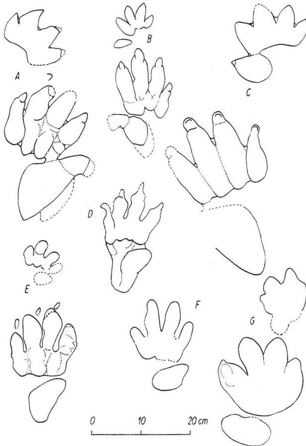
Abb. 3. Groß-Hand Chirotherien: A - C. rex , nach Peabody; B - C. barthii ; C - C. moquinense , nach Peabody. Brachychirotherien: D - C. eyermanni ; E - C. parvum , beide nach Baird; F und G - C. thuringiacum (= Brachychirotherium coburgense und hassfurtense ), F - nach Rühle v. Lilienstern; G - nach v. Freyberg
