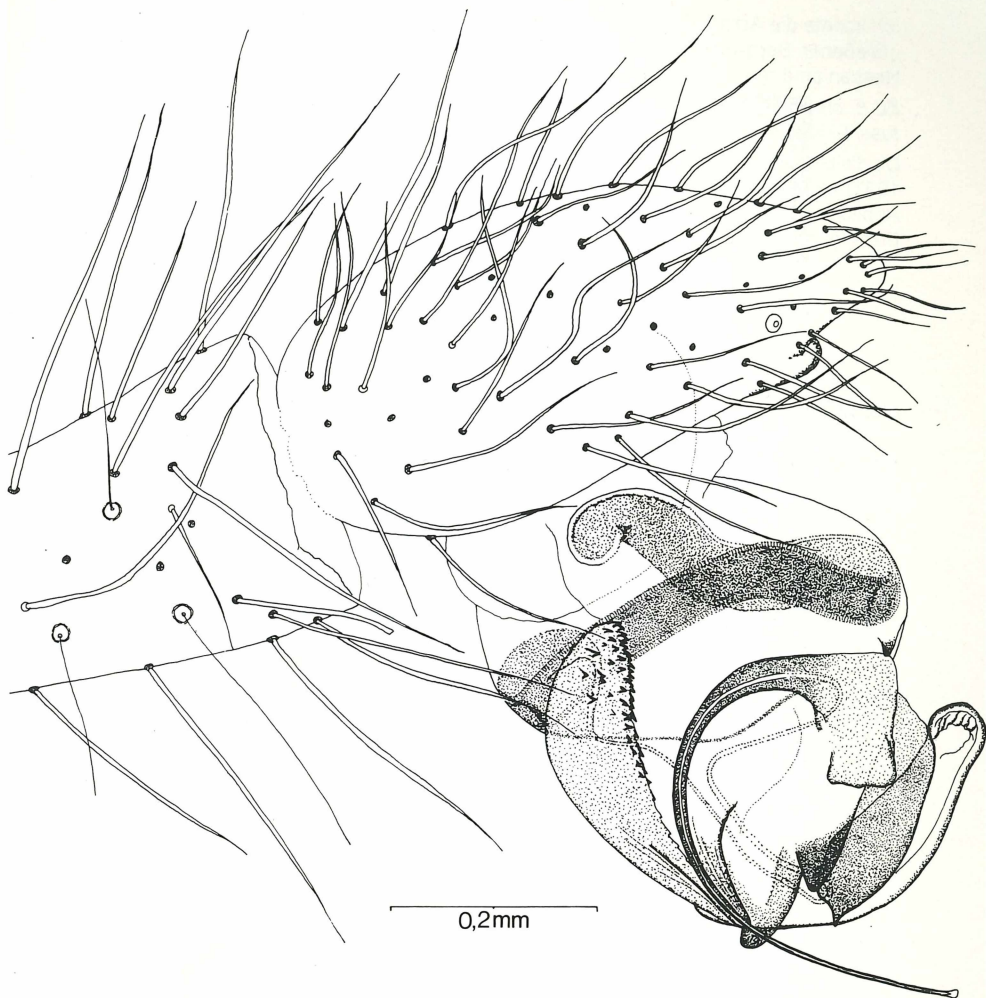
Abb. 2. Enoplognatha crucifera THORELL; Ansicht des ausgestülpten männlichen Tasters nach einem Kalilaugepräparat.
