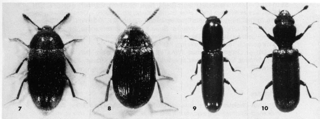
Abb. 7. Triphyllus bicolor (FABRICIUS), Länge: 3,6 mm. – Abb. 8. Mycetophagus ater (REITTER), Länge: 4,4 mm. – Abb. 9. Teredus cylindricus (OLIVIER), Länge: 4,5 mm. – Abb. 10. Lyctus brunneus (STEPHENS), Länge: 4,1 mm.
