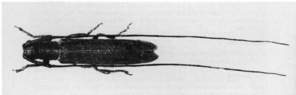
Abb. 15. Calamobius filum (ROSSI), Länge (ohne Fühler): 8,3 mm.
