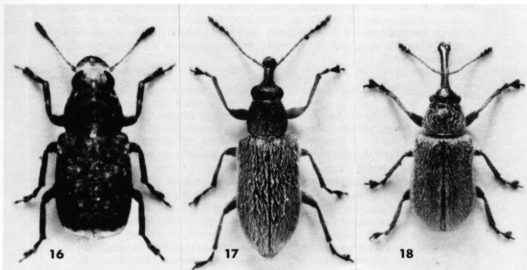
Abb. 16. Dissoleucas niveirostris (FABRICIUS), Länge: 4,7 mm. – Abb. 17. Rhinomacer attelaboides FABRICIUS, Länge: 5,3 mm. – Abb. 18. Doydirhynchus austriacus (OLIVIER), Länge: 5,0 mm. Alle Fotos: H. KRETSCHMER
