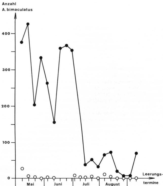
Abb. 14. Populationsentwicklung von Anthicus bimaculatus (ILLIGER) auf zwei nur durch einen Sandweg getrennten Spargelfeldern bei Pfungstadt, 1986 (s. a. RETHMEYER 1987); ● = Feld I, ○ = Feld II. Fänge mit 8 bzw. 10 Bodenfallen von etwa 10 cm Durchmesser. Die Anzahl gefangener Tiere ist gegen die wöchentlichen Leerungstermine der Fallen aufgetragen.
