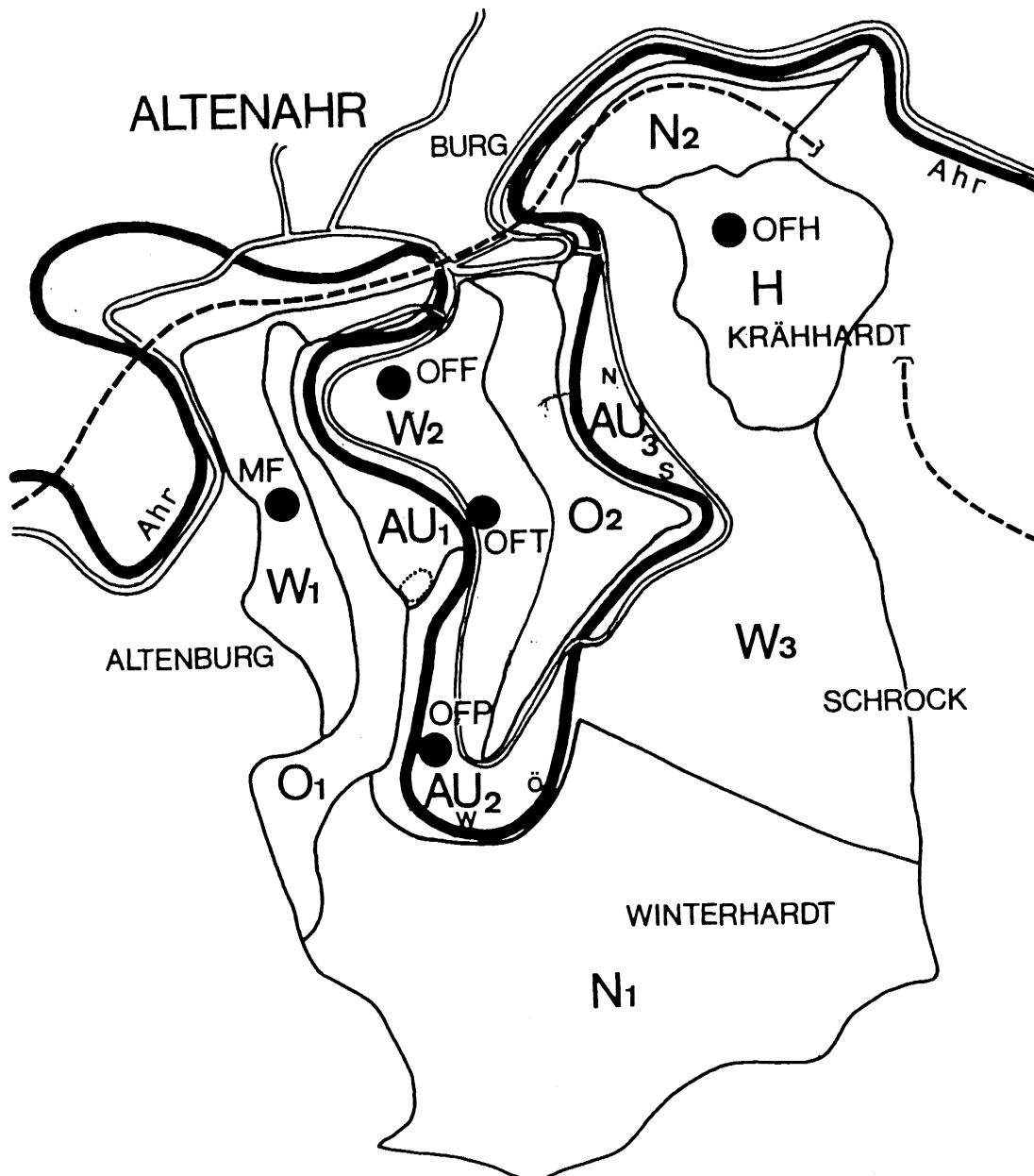
Abb. 3.6/1: Skizze des Untersuchungsgebietes NSG "Ahrschleife bei Altenahr" mit eingezeichneten Untersuchungsflächen und Fallenstandorten. Abkürzungen: MF = Malaise-Falle; OF,F, OF,H, OF,P, OF,T = Oliver-Fallen F, H, P und T; AU 1-3 = Flußniederung, AU 2W/2Ö = westliche/östliche Hälfte, AU 3N/3S = nördliche/südliche Hälfte; H = Krähhardt, N 2 = Gebiet nördl. Weinbergshang; übrige Beschriftung s. BÜCHS (1993).
