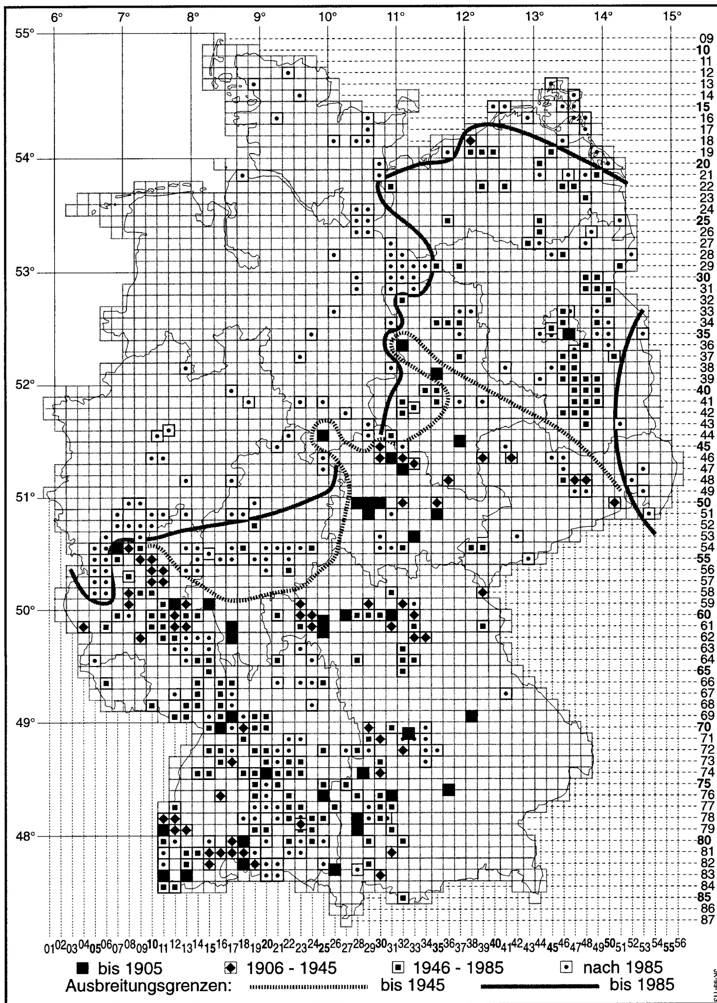
Abb. 1 : Fundnachweise und Ausbreitung von Graphosoma lineatum (LINNAEUS, 1758) Quadrate = Top. Karten 1: 25 000.
