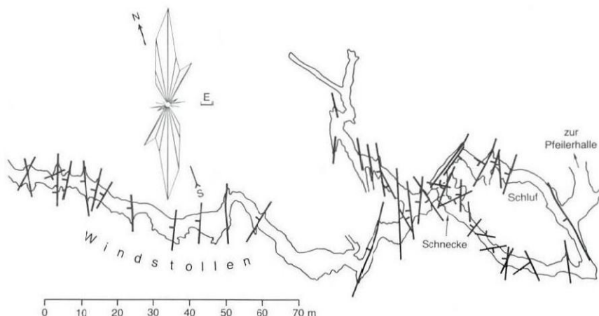
Abb. 6: Streichen und Fallen der Verwerfungen im Windstollen, in der Schnecke und im Schluf (Einnessung: E. Arnberger und E. Zirkl). Wiedergabe nicht genordet. Konstruktion des Kluftdiagramms wie bei den Abb. 4 und 5.
