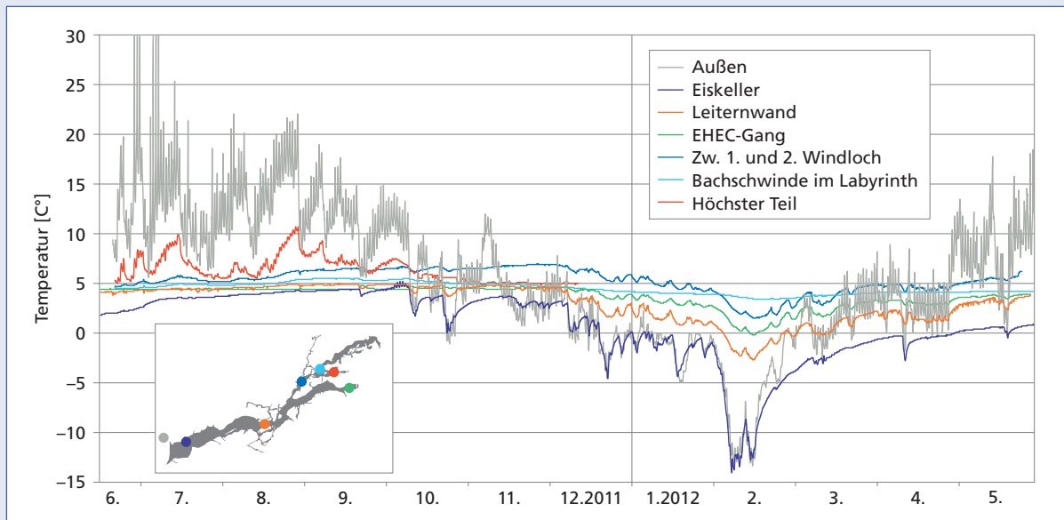
Abb. 13: Der von Datensammlern aufgezeichnete Lufttemperaturverlauf im Schneckenloch zwischen 14.6.2011 und 27.5.2012. Fig. 13: Air temperature in Schneckenloch recorded by data loggers between June 14, 2011 and May 27, 2012.
