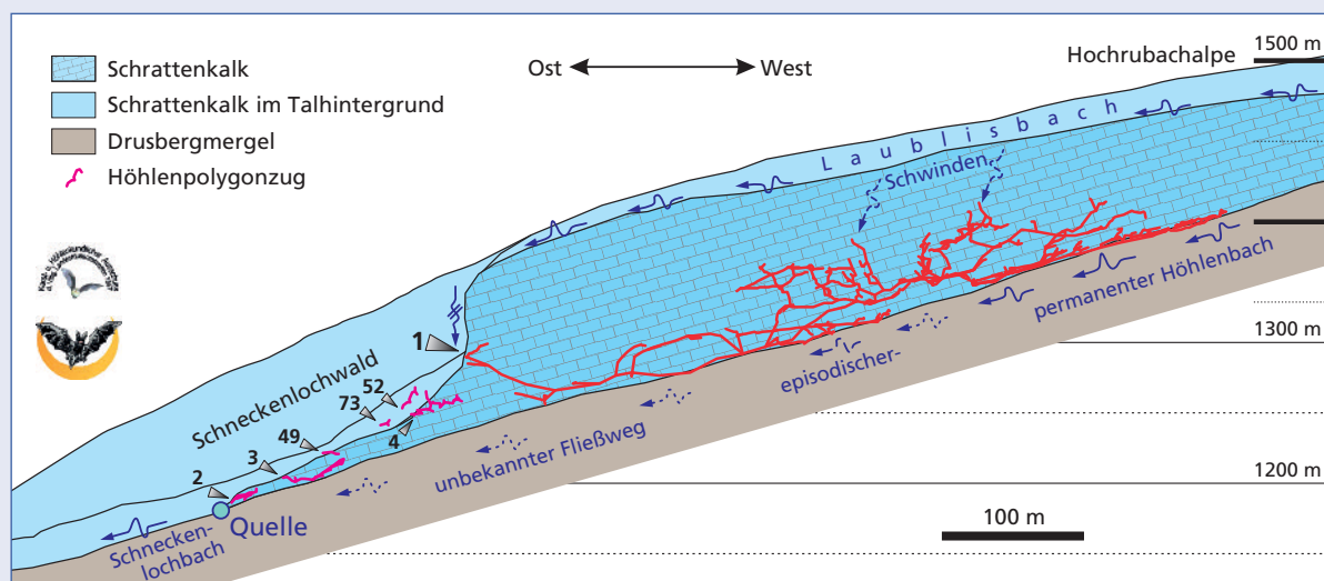
Abb. 10: Schematischer Schnitt durch das Schneckenloch. Gut ersichtlich sind die teilweise sehr geringe Überlagerung von nur wenigen Zehnermetern sowie die Anlage der Höhle an der Gesteinsgrenze.
