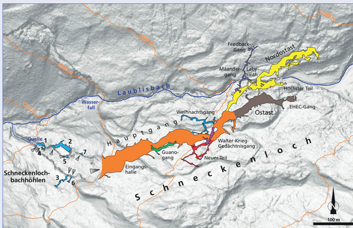
Abb. 3: Übersichtsplan des Schneckenlochs. Farblich unterschieden sind die im Text erwähnten bedeutenden Höhlenteile. Hintergrund: Schattiertes Höhenmodell (VOGIS – Land Vorarlberg).
