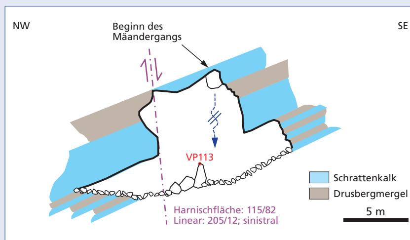
Abb. 11: NW-SE-Profil im Raum zwischen I. und II. Windloch, wo eine markante Störung die Schichten am Übergang von Drusbergmergeln und Schratenkalk versetzt.
