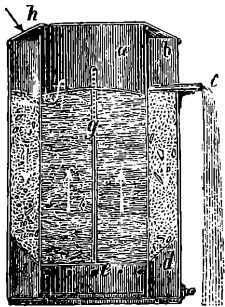
Filter-Apparat aus Zinnblech.
