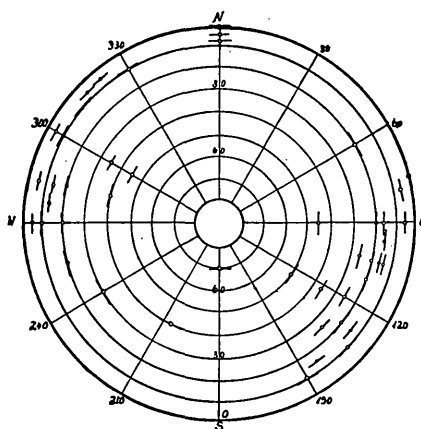
Abb. 2. Stereographische Projektion der Hauptklüfte und Kluftscharen der D. R. E. auf die Horizontale (Darstellung nach Salomon u. O. Seitz). Man erkennt deutlich ein Hauptkluftstreichen NE — SW, ein Nebenkluftstreichen NW — SE und das steile Fallen der meisten Klüfte in Richtung SE und NW.
