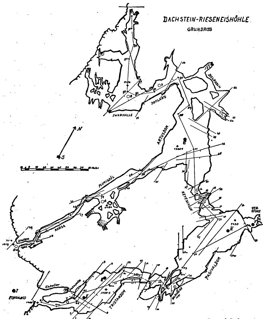
Abb. 1. Eingezeichnet sind die meteorologischen Meßpunkte (St.) ● I, II, usw., Autographenstationen; ○ 1, 2 usw., Standthermometer und Fels temperatur-Meßstellen; weiter der Verlauf der wichtigsten Klüfte, Kluftscharen (Verwerfer), der Hauptpolygonzug und die wichtigsten Höhenknoten.
