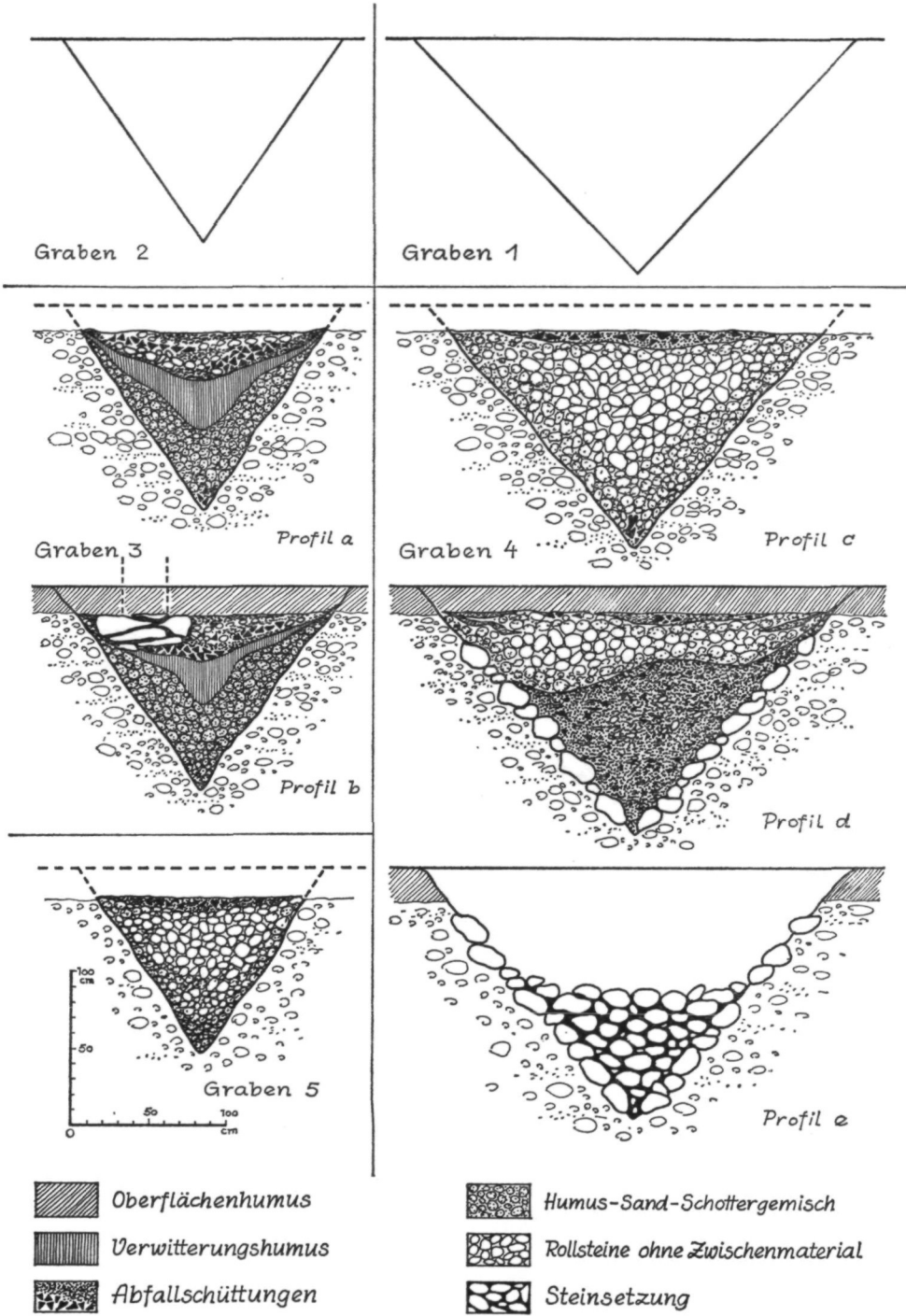
Textabb. 3: Querprofile der Spitzgräben 1—5.
