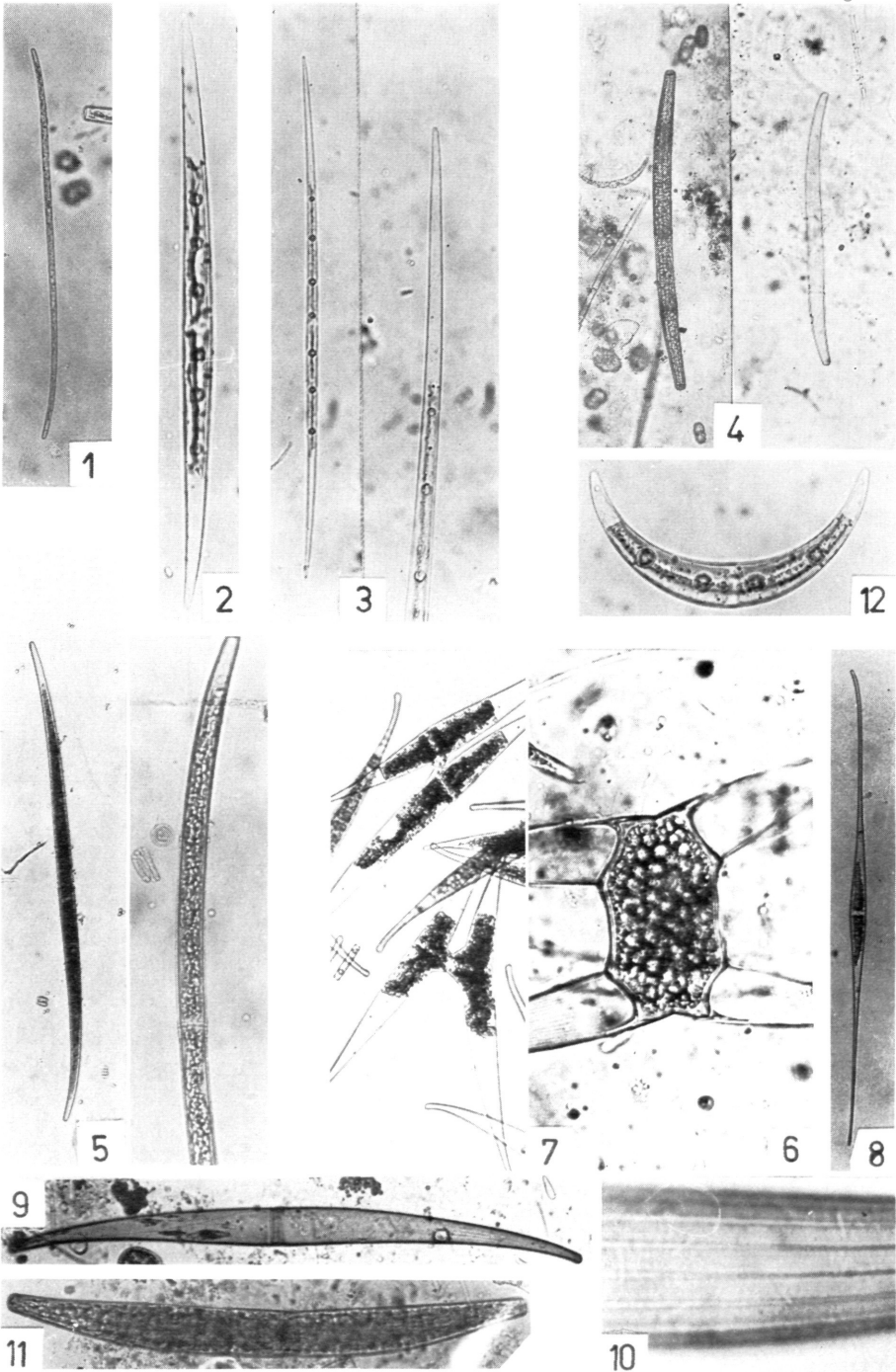
Fig. 1: Closterium lineatum (100fache Vergr.). – Fig. 2: Closterium idiosporum (300fache Vergr.). – Fig. 3: Closterium pronum – Gesamtansicht (100fache Vergr.) und Zelle (300fache Vergr.). – Fig. 4: Closterium juncidum (100fache Vergr.). – Fig. 5: Closterium lineatum – Gesamtansicht (100fache Vergr.) und Zelle (300fache Vergr.). – Fig. 6: Konjugierende Zellen von Clost. rostratum (100fache Vergr.). – Fig. 7: Zygote von Clost. rostratum (300fache Vergr.). – Fig. 8: Closterium setaceum (50fache Vergr.). – Fig. 9: Closterium Ralfsii var. hybridum (30fache Vergr.). – Fig. 10: Zellhautstruktur von Clost. costatum (600fache Vergr.). Fig. 11: Closterium striolatum (150fache Vergr.). – Fig. 12: Closterium parvulum (600fache Vergr.).
