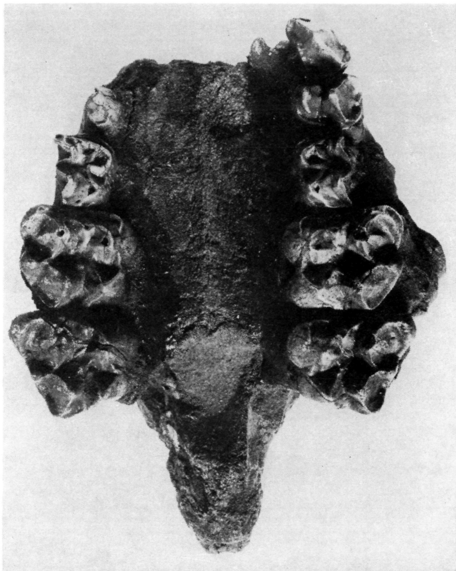
Abb. 3: Die Schädelbasis von Anthracotherium frehi n. sp. aus den älteren Linzer Sanden der Reisetbauer-Sandgrube bei Alharting. \frac{4}{5} der nat. Größe.
