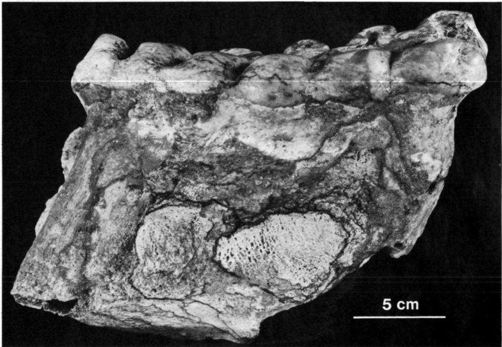
Abb. 4: Tetralophodon longirostris (KAUP), M 3 inf. dext. von buccal (labial).
