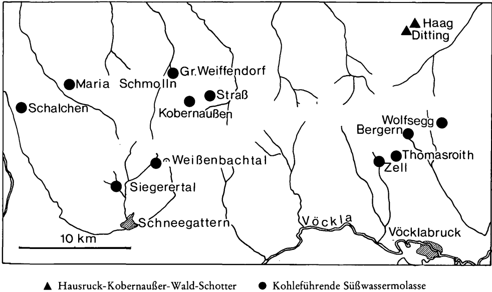
Textabb. 2: Fundortskizze jungtertiärer Vertebratenreste aus dem Hausruck- und Kobernauber Wald (siehe Tab. 1).
