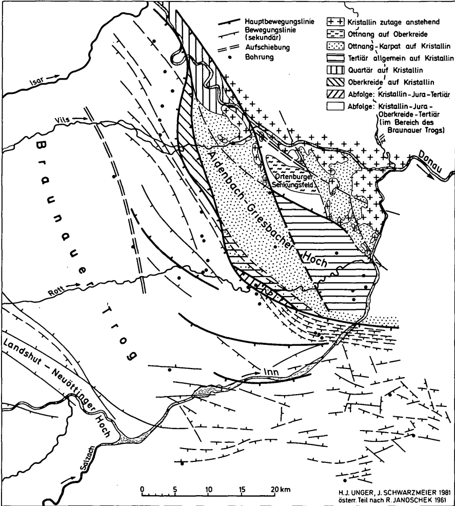
Abb. 3: Räumliche Darstellung der verschiedenen Schichtenabfolgen in Ostniederbayern
