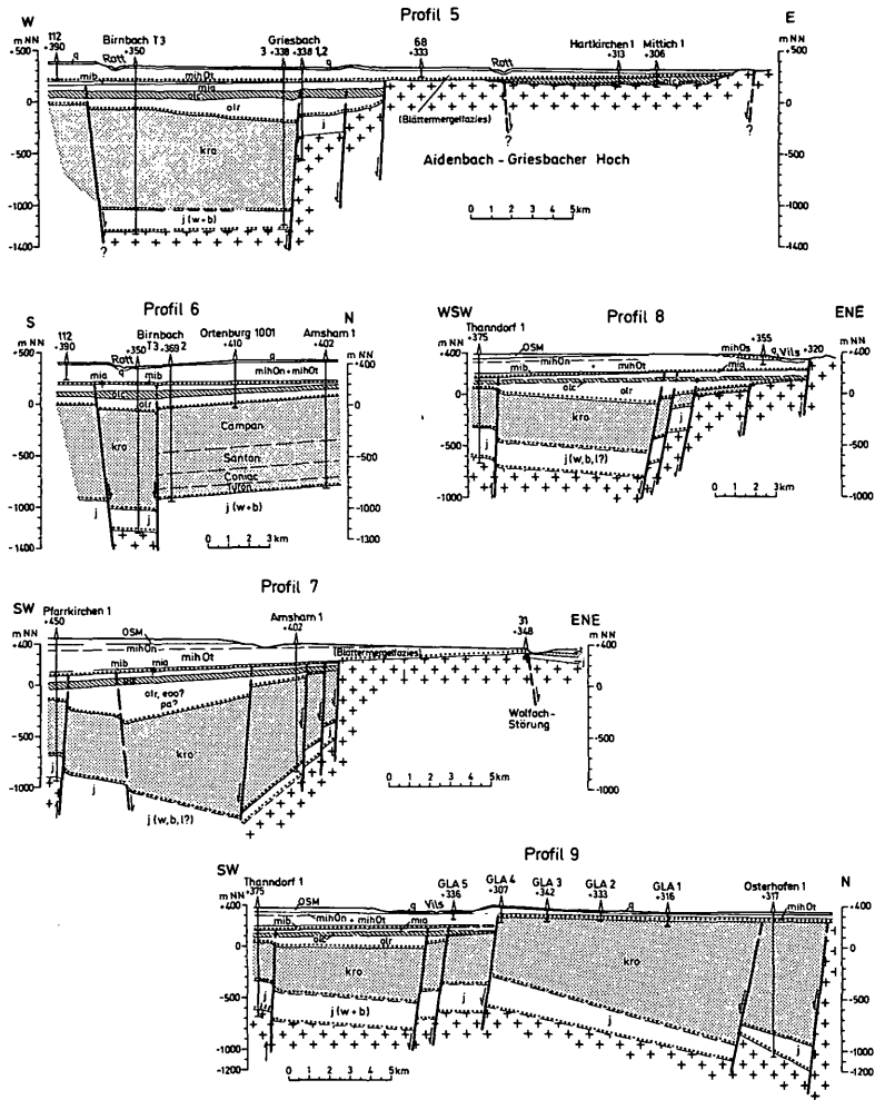
Darstellung nach E. KRAUS 1915, H. NATHAN 1949, F. OSCHMANN 1954, R. JANOSCHEK 1961, H. GUDDEN u. J. H. ZIEGLER 1965, M. BAUMANN, W. REGNET u. P. UDLUFT 1975 u. F. X. FÜHRER 1978 H. J. UNGER u. J. SCHWARZMEIER 1981
