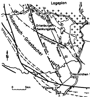
Abb. 9: Tektonische Entwicklung und geologischer Werdegang des ostniederbayerischen Raumes (Tertiär bis Quartär)
