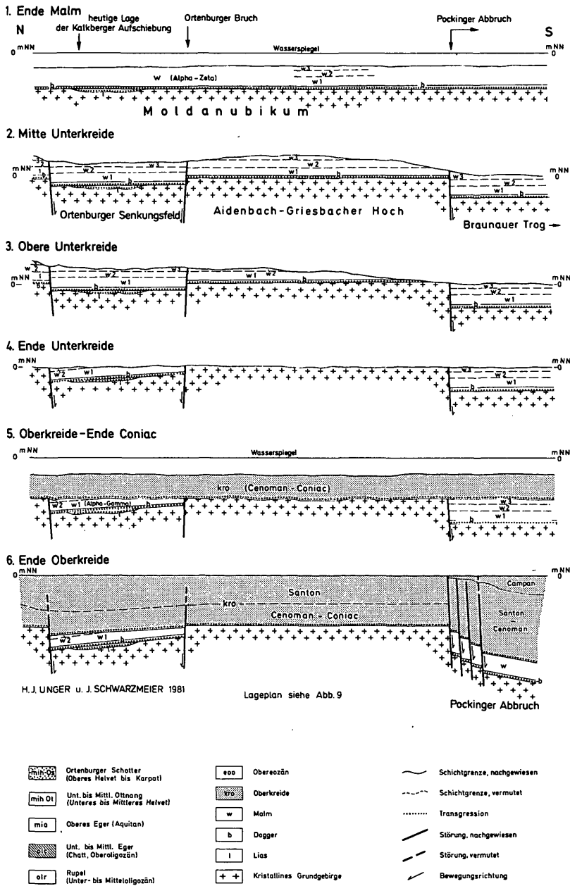
Abb. 8: Tektonische Entwicklung und geologischer Werdegang des ostniederbayerischen Raumes (Jura bis Kreide)
