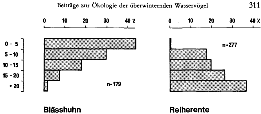
Abb. 15: Aufenthaltsbereiche für Blässhuhn und Reiherente – links: Entfernung vom Ufer.
