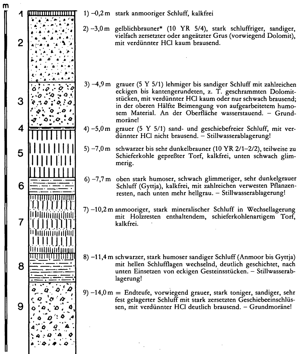
Abb. 2: Sedimentfolge Bohrung 259 – siehe nebenstehende Beschreibung.
