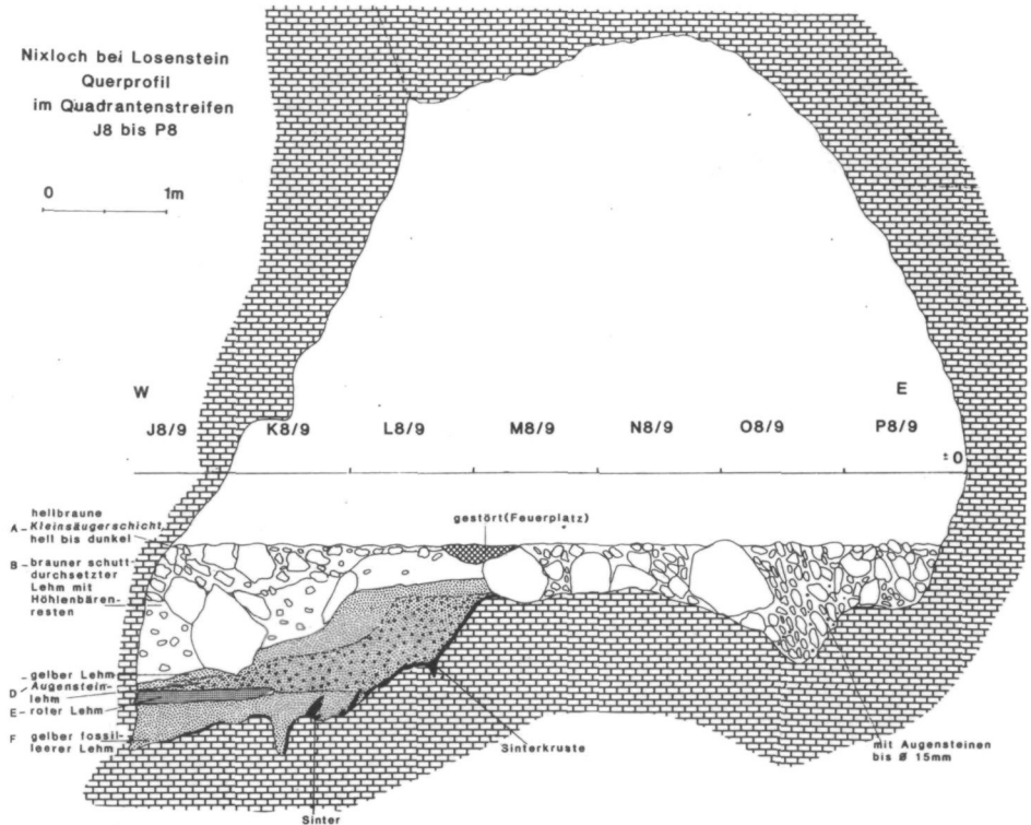
Abb. 3: Querprofil an den Quadrantengrenzen 8/9.
