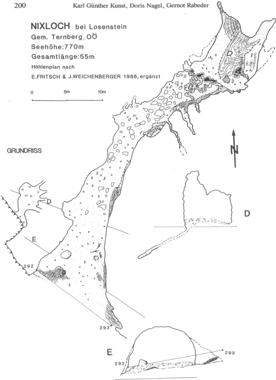
Abb. 1: Höhlenplan — Grundriß und Querprofile.
