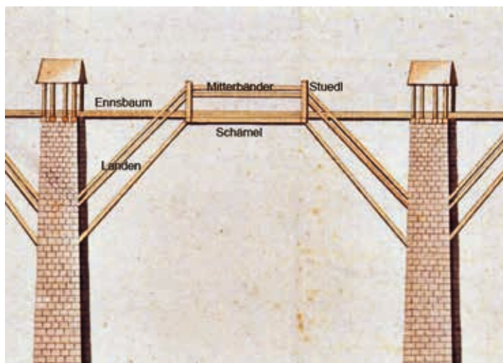
Abb. 50: Detail Spannwerk des Gosauzwangs (Finanz- und Hofkammerarchiv Wien – Öst. Staatsarchiv, Sign. H 112).
