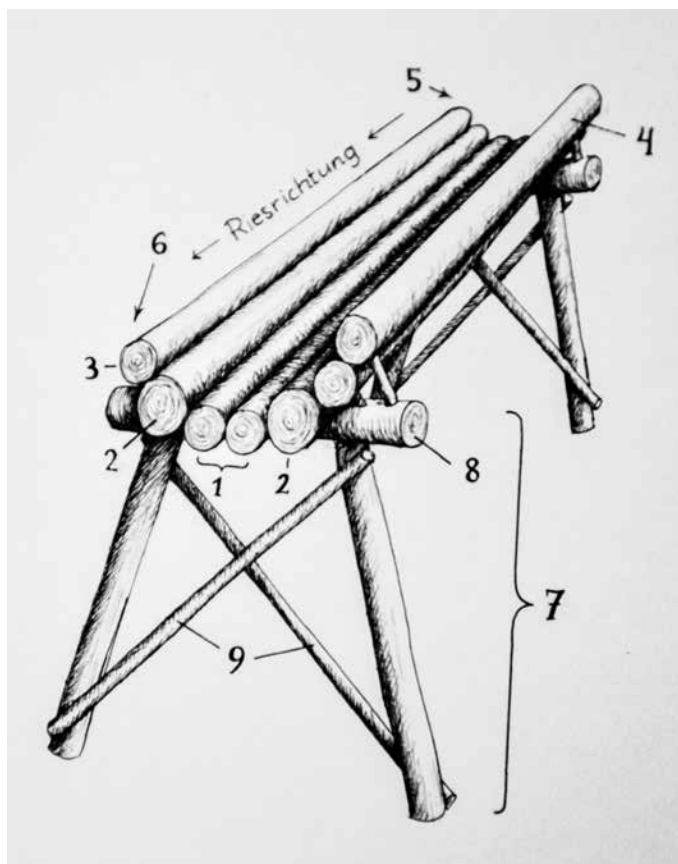
Abb. 48: Holzries (Zeichnung: Kurt Druckenthauer 2007). 167
