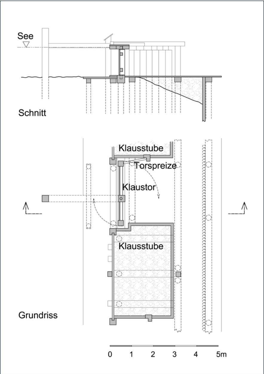
Abb. 66: Grundriss und Schnitt eines Klaustores (Planzeichnung des Autors).
