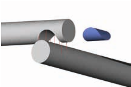
Abb. 59: Axonometrie Rundholzecke (Zeichnung: Idam).
