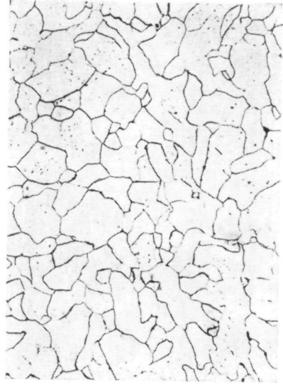
Bild 4: Römisches Eisenmesser, ferritische Grundmasse. Ätzung: Alkoholische Salpetersäure. Vergrößerung: 70fach.
