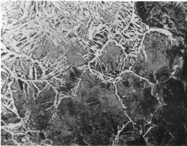
Bild 5: Römisches Eisenmesser. Rechts und unten aufgekohlte Randzone (Zementitnetzwerk, dazwischen Perlit); nach links oben abfallender Kohlenstoffgehalt und Übergang zu reinferritischem Gefüge (wie in Bild 4 gezeigt). Ätzung: Alkoholische Salpetersäure. Vergrößerung: 100fach.
