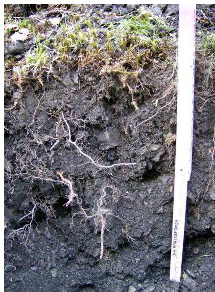
Abb. 15: Regosol aus Bergematerial auf einer Brachfläche der Zeche Bismarck in Gelsenkirchen (2007, T. KASIELKE).
