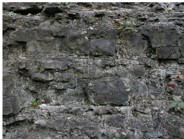
Abb. 30: Geschichtete Schlacken im Landschaftspark Duisburg-Nord (2010, C. BUCH).
