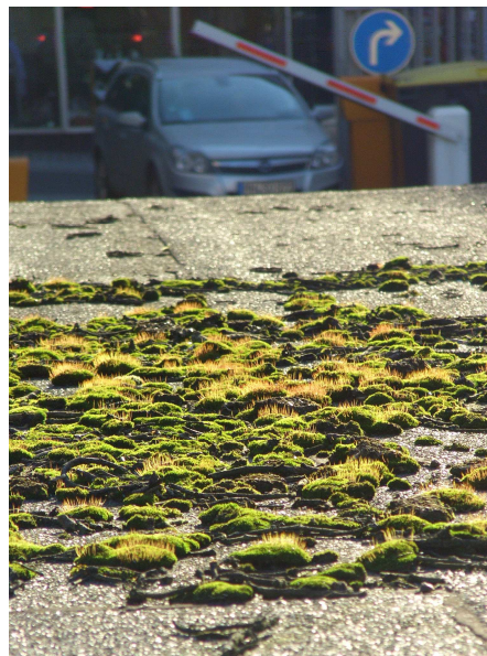
Abb. 11: 'Felshumusboden' aus Moos auf einem Flachdach in der Mülheimer Innenstadt (2010, T. KASIELKE).
