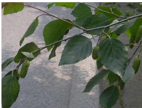
Abb. 4: Die im Aachener Raum recht häufige Betula ×aurata ähnelt von der Blattform her B. pubescens s. str. Betula ×aurata , which is quite frequent in the region of Aachen, resembles B. pubescens s. str. in leaf shape. Bleiberger Straße, Aachen/NRW (14.06.2006, F. W. BOMBLE).
