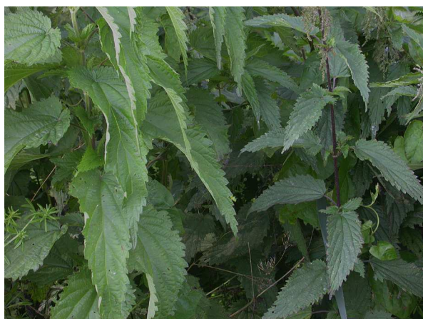
Abb. 12: Urtica subinermis (links) und U. dioica s. str. (rechts). Urtica subinermis (left) and U. dioica s. str. (right). Zwischen Bienen und Grietherbusch, Kreis Kleve/NRW (26.06.2004, F. W. BOMBLE).
