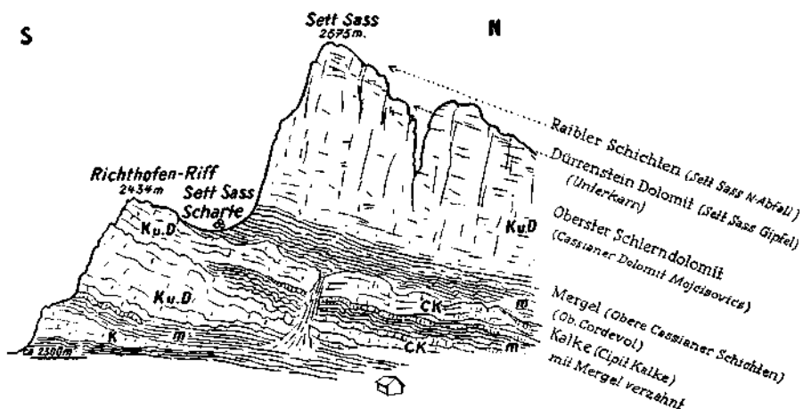
Textabbildung 3: Ostansicht des Richtshofen-Riffs (nach Ogilvie Gordon 1929, ergänzt nach G. Rosenberg 1959). Verzahnung der Cassianer Mergel (m) und Kalke (K) mit auskeilenden Riffmassen von Kalk und Dolomit (K und D), die zum Teil in Cipitkalk (CK) übergehen.
