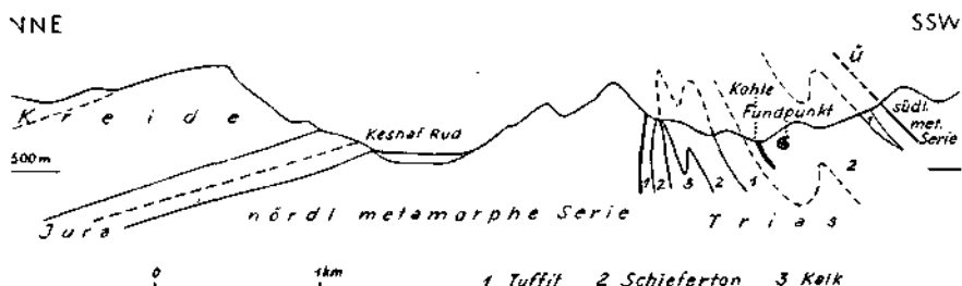
SAMMELPROFIL nach K. T. Goldschmid und A. Rutner Textabbildung 4: Der Fossilfundpunkt bei Aghdarband (Nordostpersien).
