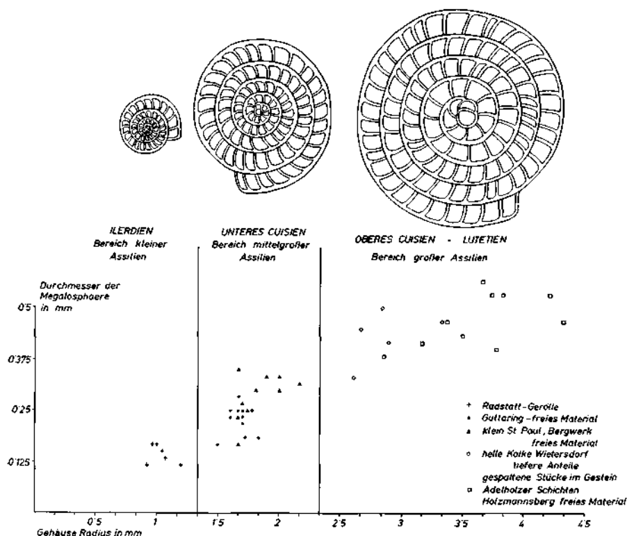
Abb. 10. Übersicht von Medianschnitten kleiner, mittelgroßer und großer Assilien. Das Diagramm gibt das Verhältnis von Durchmesser der Megalosphäre und Radius aus verschiedenen Vorkommen, um die Möglichkeiten einer biostratigraphischen Auswertung geringen Materials zu veranschaulichen.
