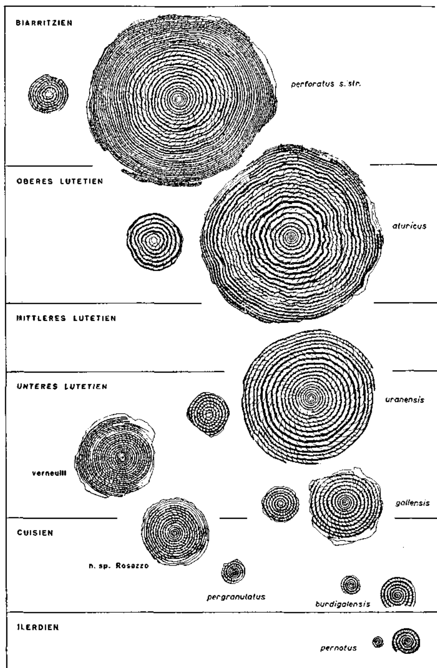
Abb. 7. Evolution der Nummuliten aus der Gruppe des N. perforatus , die starke Größenzunahme vom Ilerdien zum Lutetien verdeutlichend. Aus H. SCHAUB, 1963, übernommen, Medianschnitte.
