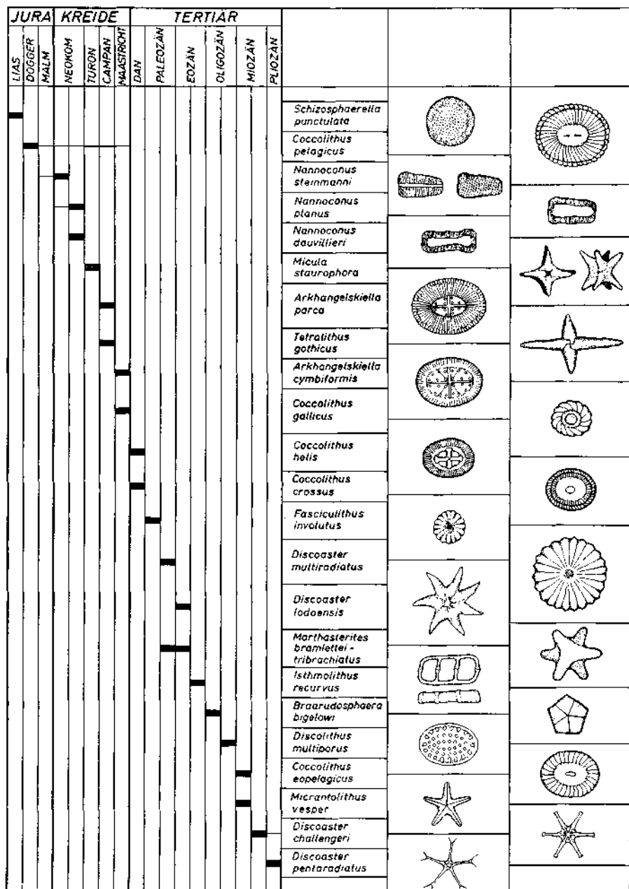
Abb. 2. Übersicht leitender Nannofossilien.
