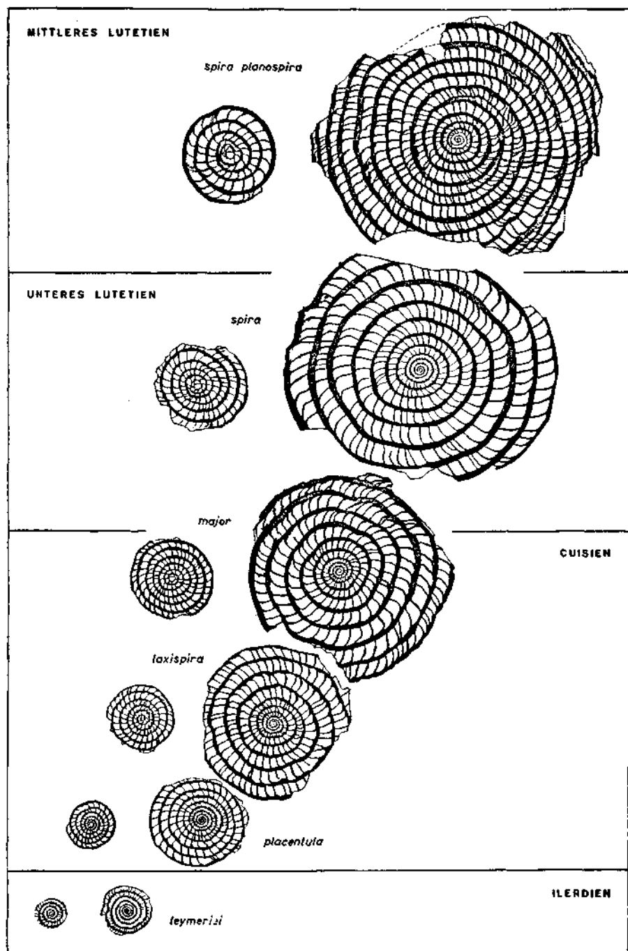
Abb. 8. Evolution der Assilinen aus der Gruppe der Assilina spira , die starke Größenzunahme vom Ilerdien zum mittleren Lutetien zeigend, Medianschnitte. Aus H. SCHAUB, 1963, übernommen.
