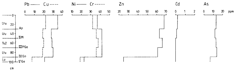
Abb. 5. Tiefenverteilung der Schwermetalle in einem Auenpelosol-(Brauner) Auenboden aus verschiedenen Hochflutlehmen über Auensand (Beprobungspunkt 10, R: 346138, H: 551093).
