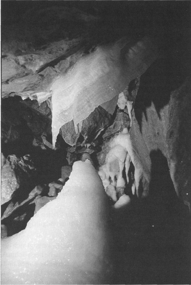
Abb. 2: Sinterfahne und Makkaronis im Eingangsbereich der Herbstlabyrinth-Höhle („Willy-Hofmann-Halle“) (Foto: C. GRUBERT).
