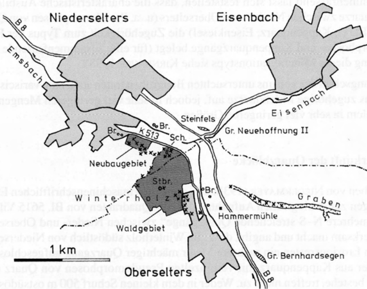
Abbildung 1: Fundstellen der Pseudomorphen- und Kappenquarzblöcke bei Nieder- und Oberselters (Kreuzsignatur). Die Mineralwasserbrunnen und -bohrungen (Br.) beider Ortschaften sind als offene Kreise dargestellt. Stbr. = Steinbruch, Sch. = Schurf
