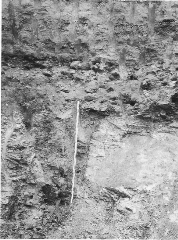
Abbildung 4: Steil stehender Basaltgang (Eozän) durchschlägt Serizitgneis (Silur) und wird selbst von jüngeren Sedimenten (Oligozän) gekappt (SSE-Ecke Baugrube Kapellenstraße/Wiesbaden)
