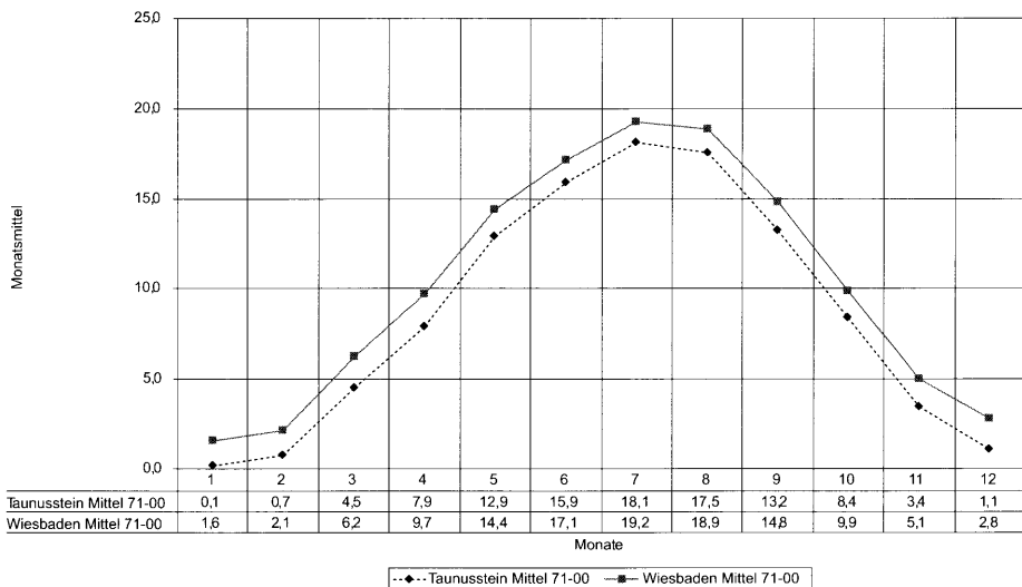
Abbildung 2: Klimadiagramm der Monatsmitteltemperaturen Wiesbaden und Tausstein 1971 bis 2000
