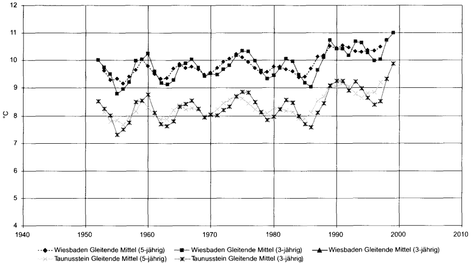
Abbildung 7: Gleitende Mittel der Lufttemperaturen Wiesbaden und Taunusstein 1951 bis 2000
