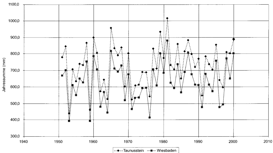
Abbildung 3: Jahressummen Niederschlag Wiesbaden und Tausstein 1951 bis 2000
