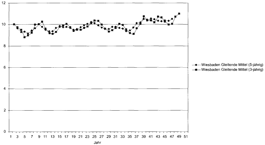
Abbildung 5: Gleitende Temperatur-F-Mittel Wiesbaden (1951–2000)
