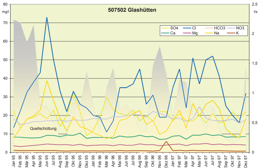
Abbildung 7: Konzentration (in mg/l) ausgewählter Inhaltsstoffe im Grundwasser der Messstelle 507502 Glashütten sowie mittlere monatliche Quellschüttung im Zeitraum 1995 - 1997.
