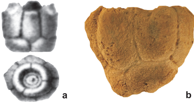
Abbildung 1: a-b. ?Hexacrinites brevis (GOLDFUSS 1839).
