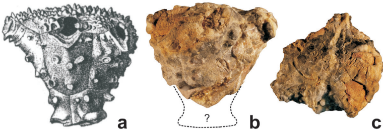
Abbildung 5: a. ? Hexacrinites spinosus (MÜLLER 1856); b-c. ? H. cf. spinosus (MÜLLER 1856). a. Holotypus (Nr. MCZ-103054) nach MÜLLER (1856); Scan der Lithographie aus SCHULTZE (1866: Taf. 8, Fig. 2e); Lateralansicht des B-Radius (Grenzbereich Eifelium/Givetium der Prümer Mulde, Eifel) – x 1,1. b-c. Aboralkelch (Nr. CR.L.-1, Slg. LEUNISSEN); b. Lateralansicht des B-Radius (Mittel-Givetium von Villmar) – x 0,8. c. Wie b; Oralansicht – x 0,7.
