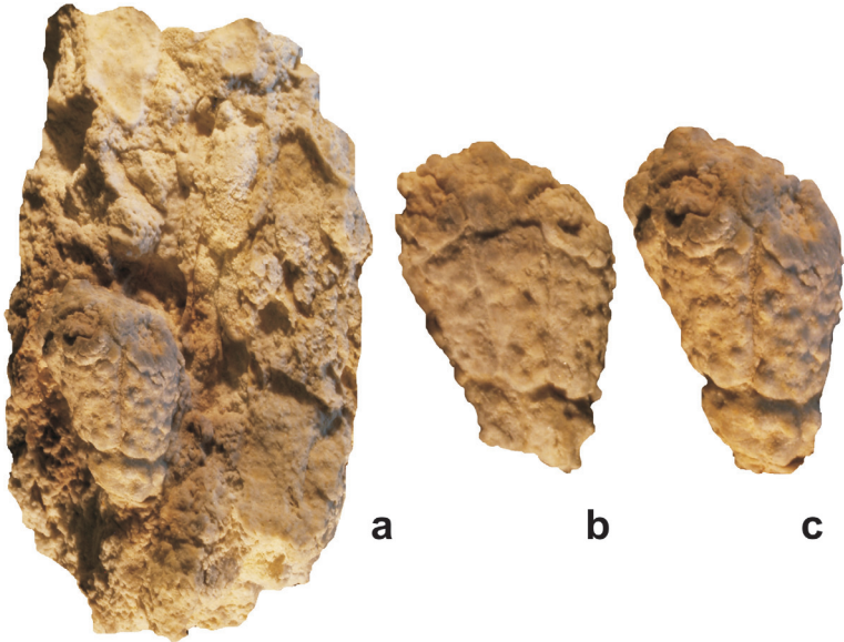
Abbildung 7: a-c. ?Hexacrinites heidelbergi n. sp.
