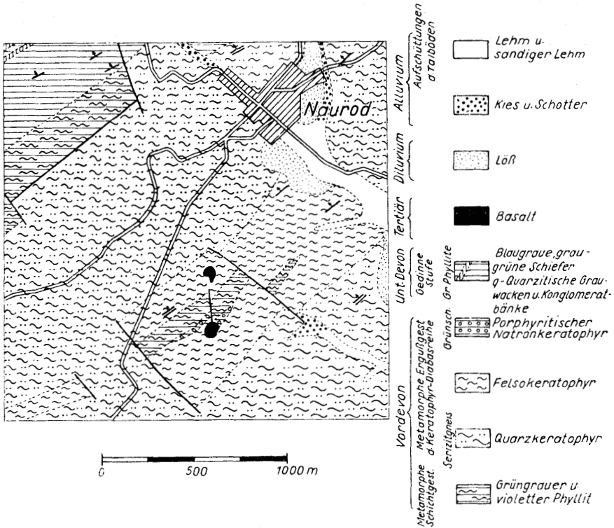
Abb. 2. Ausschnitt aus der geol. Karte Preußen u. ben. deutsche Ländern, Blatt Wehen (Lieferung 288).
