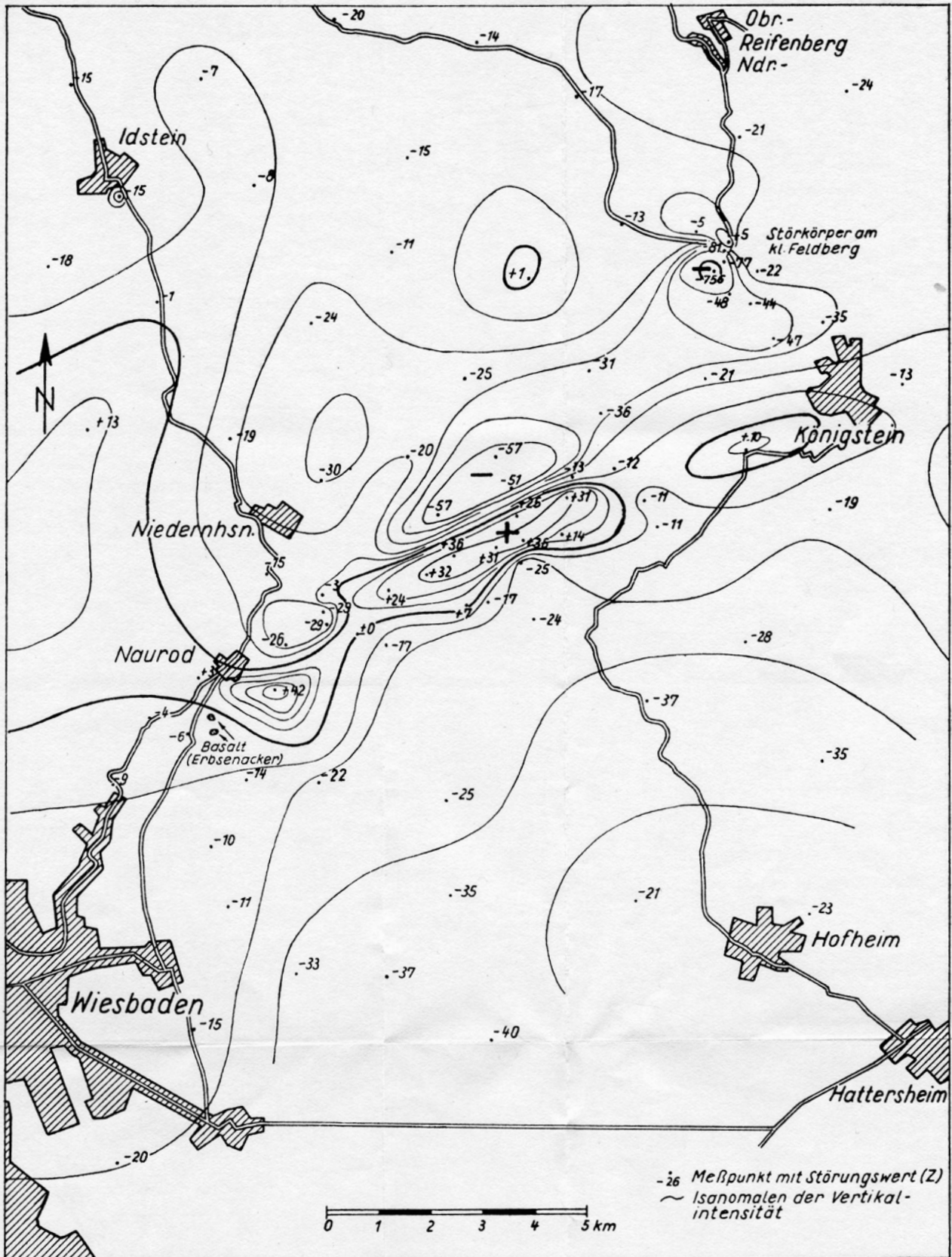
Abb. 6. Isanomalienkarte (Z) des südlichen Taunusgebietes zwischen Wiesbaden und Königstein. Nach unveröffentlichten Messungen von H. REICH.
