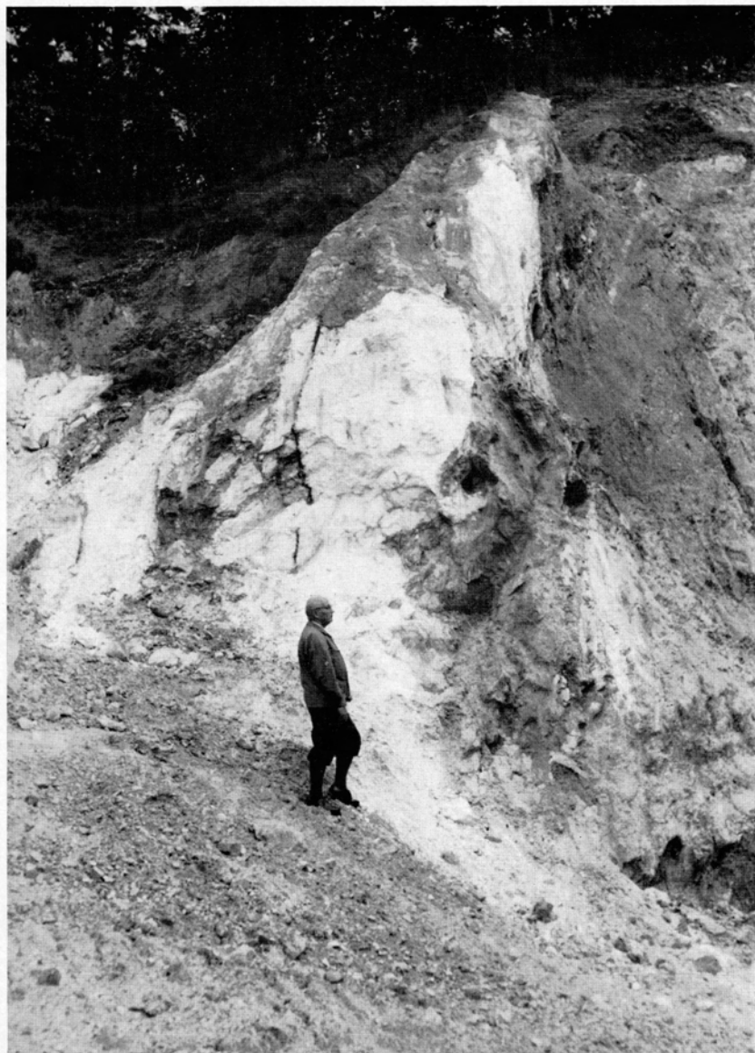
Gang von weißem, feinsandigem Quarz auf dem Heidekopf, \alpha des Profils. Aufnahme des Verfassers vom 24. 9. 1960; seitdem weiter verändert.
