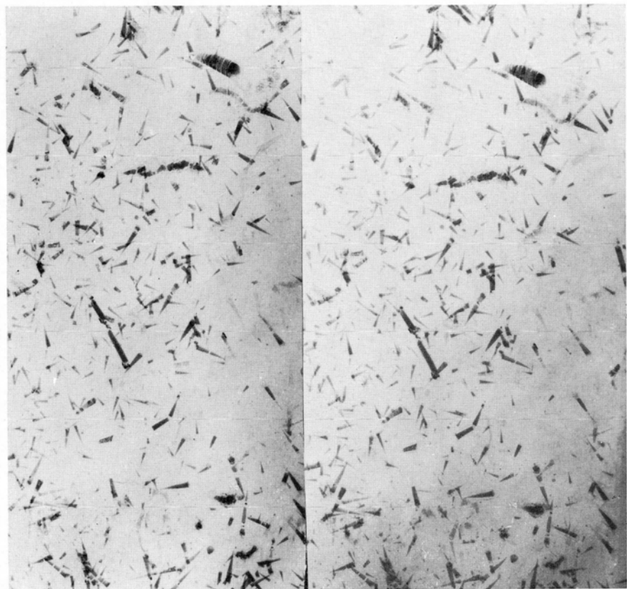
Abb. 1. Stereo-Röntgenaufnahme einer Dachschieferplatte von der Halde der Kaisergrube in Gemünden mit zahlreichen Exemplaren von Viriatellina fuchsi , weiteren fossilen Kleinformen und Detritus.
