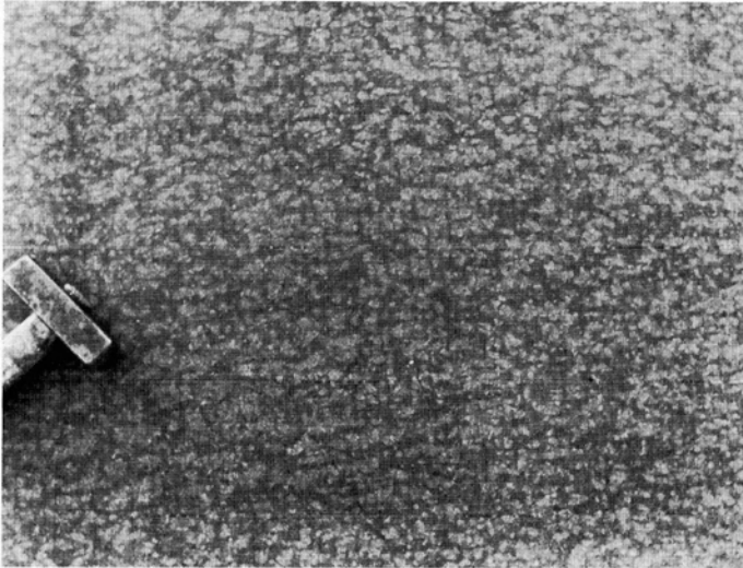
Abb. 2. Platte von Pikrit (Hirzenhain), nicht poliert mit unregelter feinkörniger Flammung. Neben der Flammung sind Kristallkörner von Pyroxen als kleine runde graue Flecke sichtbar. (Maßstab: Hammerbreite = 7 cm.)
