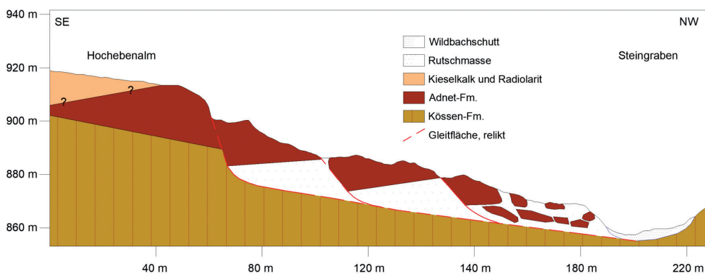
Abb. 12. Schematisches Profil durch den zentralen nördlichen Teil der Hohebenalm-Massenbewegung. Die Lage des Profils ist in Abbildung 7 ersichtlich.
