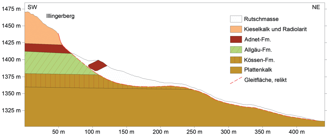
Abb. 4. Schematisches Profil durch die Massenbewegung am Illingerberg. Die Lage des Profils ist in Abbildung 3 ersichtlich.
