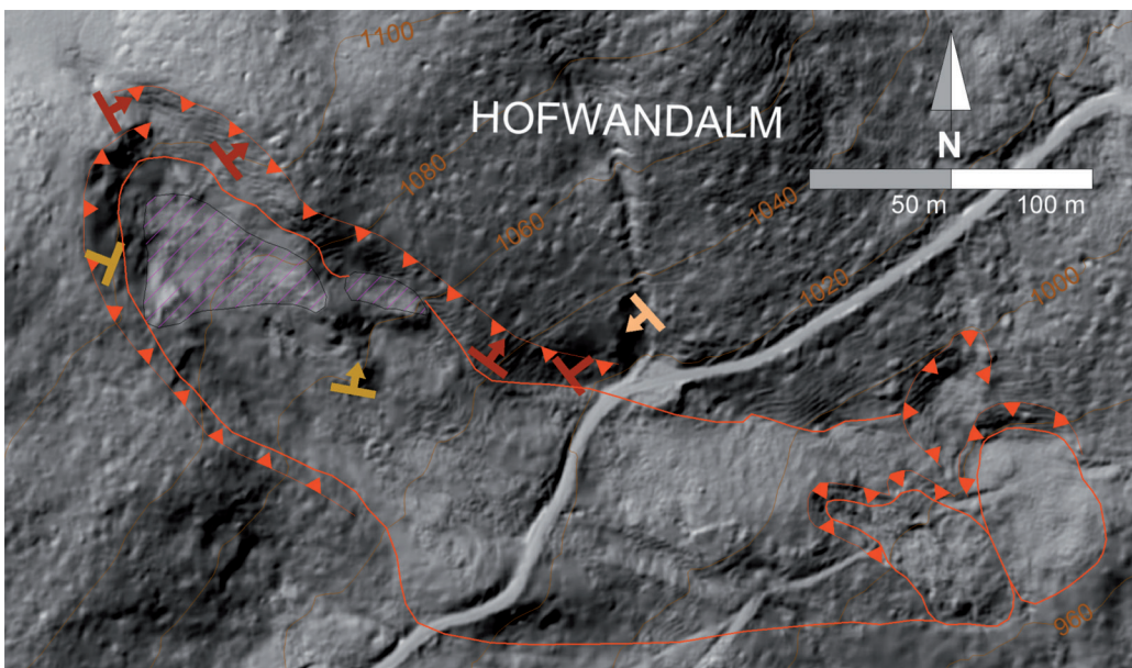
Abb. 13. Geomorphologische Übersichtskarte der Hofwandalm-Massenbewegung (5). Als topographische Grundlage dient ein digitales Geländemodell (© basemap.at).
