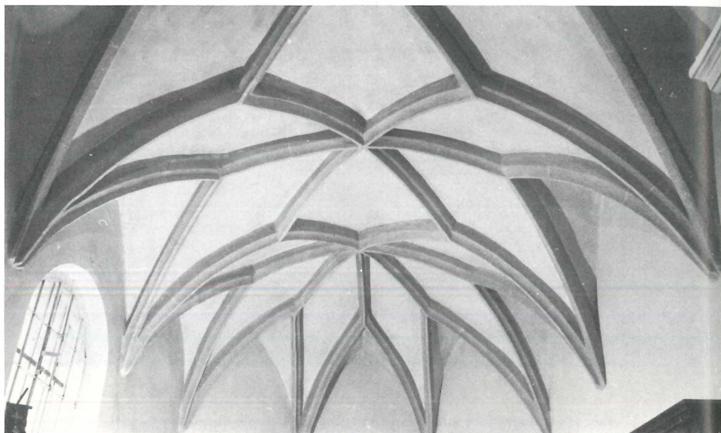
Abb. 13: Spätgotisches Gewölbe der Nordkapelle.
