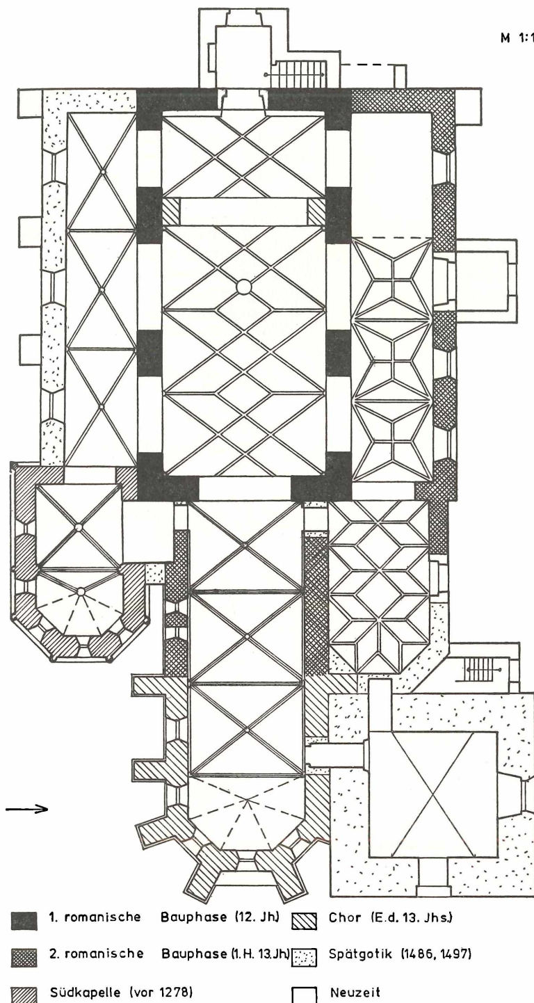
Fig. 1. Grundriß der Pfarrkirche in Großkrut, Entwurf vom Verfasser nach dem Plan von Adalbert Klaar (1953), gezeichnet von Martin Polleroß
