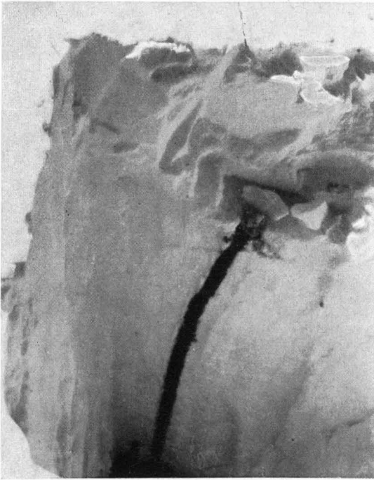
Abb. 3. Ein sogenanntes „Kriechschnee- profil“ freigelegt. Im Laufe eines Monats hat sich der ursprünglich gerade Säge- mehlstrang unter dem Einfluß des Schnee- kriechens gekrümmt. Die Abweichung von der Lotrechten ist unmittelbar über dem Erdboden gering, an der Schnee- oberfläche am größten und beträgt hier 30 cm
