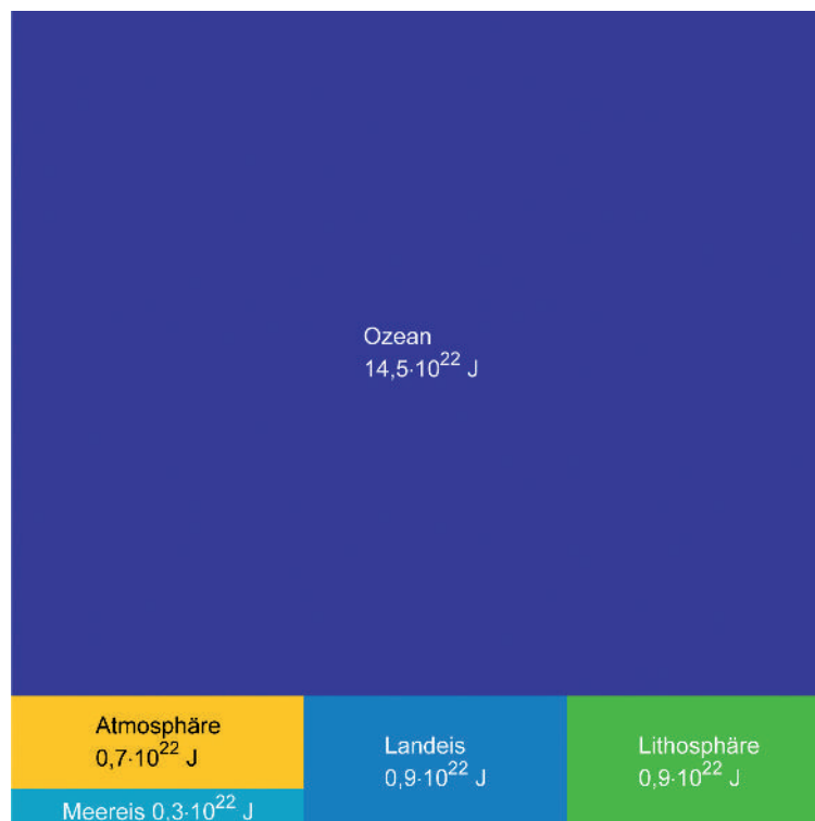
Abb. 1: Akkumuliertes planetares Energiebudget der Erde zwischen 1955 und 1998 (Daten aus LEVITUS et al., 2005). Insgesamt hat der Planet Erde in diesem Zeitraum ca. 17,3 \cdot 10^{22} J Energie aufgenommen 4 , der weitaus größte Anteil daraus ist in die Erwärmung der Ozeane gegangen. Weitere große Energiemengen wurden für die Erwärmung der Lithosphäre und das Schmelzen von Eis verbraucht. Nur etwa 5% der akkumulierten Energie spiegeln sich in der Erwärmung der Atmosphäre wieder.
