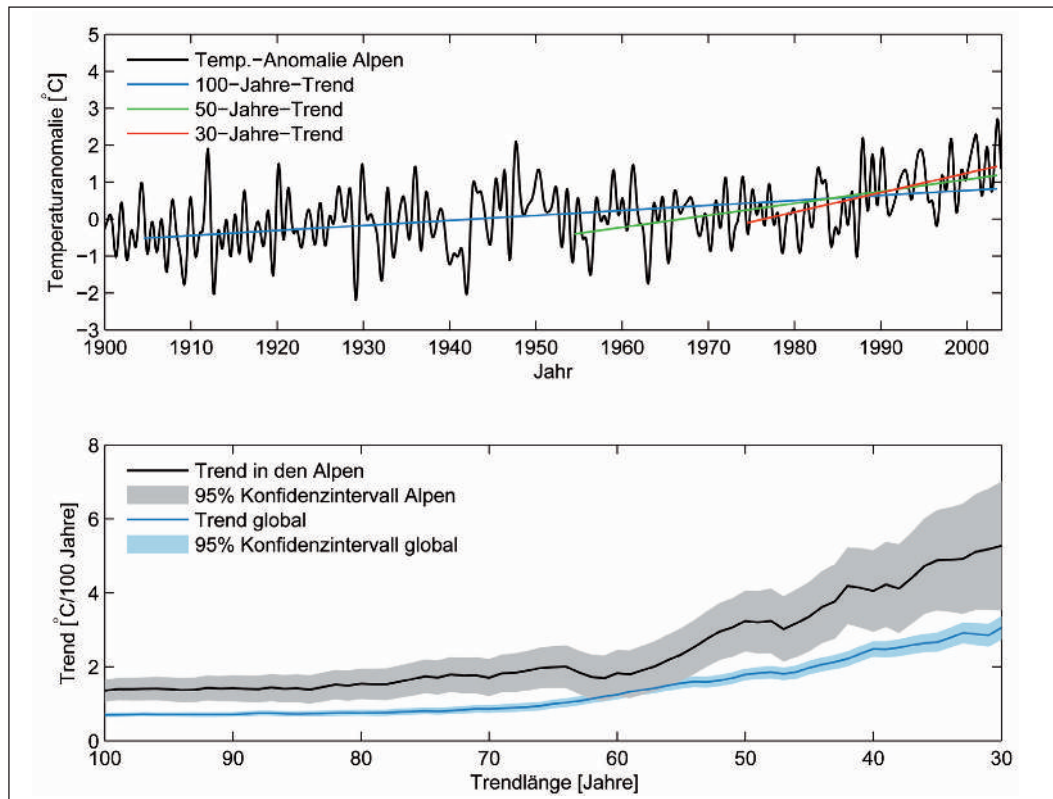
Abb. 2: Oben: Temperaturanomalien im Alpenraum seit 1900, relativ zum Temperaturmittel zwischen 1961 und 1990 (Daten aus AUER et al., 2007). Die farbigen Linien geben den linearen Temperaturtrend berechnet über die letzten 30, 50, und 100 Jahre wieder. Unten: linearer Trend der Temperaturen im Alpenraum (schwarz) und auf allen Landflächen der Erde (blau, Daten aus MITCHELL & JONES 2005), in Abhängigkeit von der Länge der Trendberechnung. D.h., die Steigung der blauen Linie im oberen Teil der Abbildung entspricht dem Wert der schwarzen Linie im unteren Teil der Abbildung bei 100 Jahren, die Steigung der grünen Linie (oben) dem Wert bei 50 Jahren (unten), und die Steigung der roten Linie (oben) dem Wert bei 30 Jahren (unten). Die Alpen folgen dem globalen Muster einer sich beschleunigenden Erwärmung, erwärmen sich aber über fast jeden Zeitraum gesehen signifikant schneller als die Welt insgesamt.
