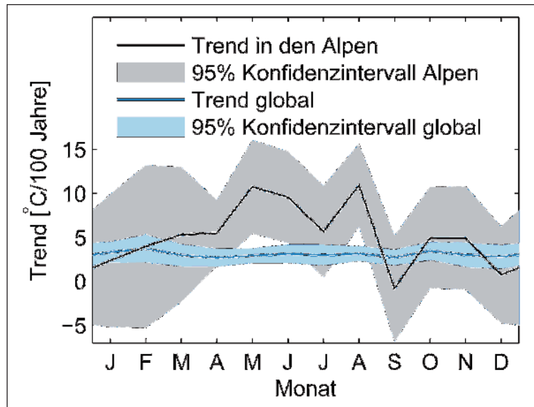
Abb. 3: Linearer, 30-jähriger Trend nach Monaten aufgeschlüsselt, schwarz: Alpenraum, blau: alle Landflächen der Erde. Die Erwärmung der Alpen ist vor allem in den Sommermonaten stärker.
