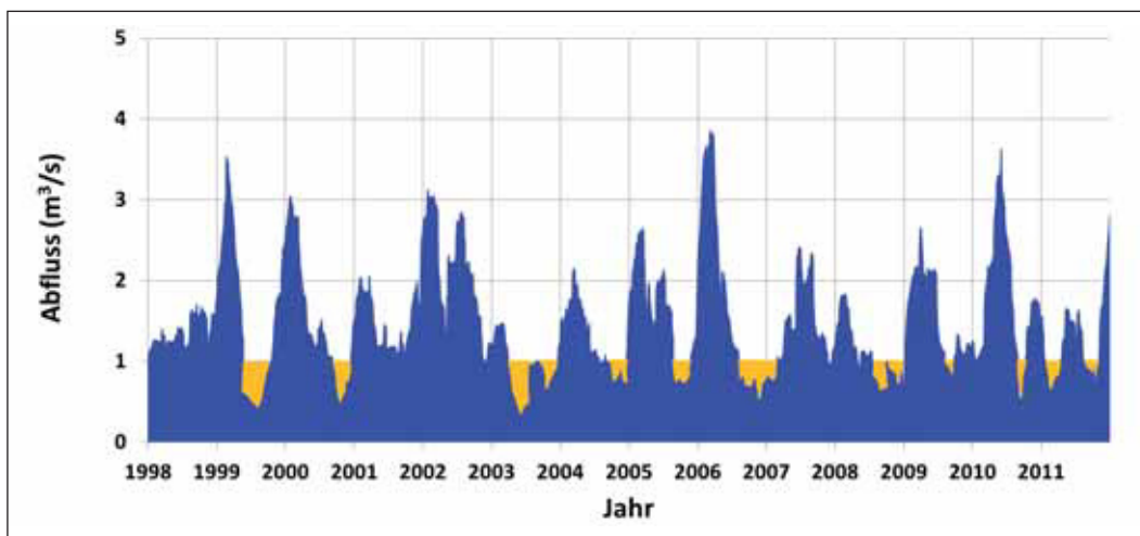
Abb. 3: Abflüsse des Auerbaches (Mangfallgebirge) bei Bad Trissl/Oberaudorf (504 m)/Oberbayern zwischen 1998 – 2011. Mittlere tägliche Abflüsse gemittelt durch den drei-monatigen gleitende Mittelwert. Die gelben Täler zeigen Zeiten mit Niedrigwasserabflüssen. Seit 1999 gibt es mit Ausnahmen in jedem Jahr ausgedehnte Phasen mit Niedrigwasser (DE JONG 2013c).
