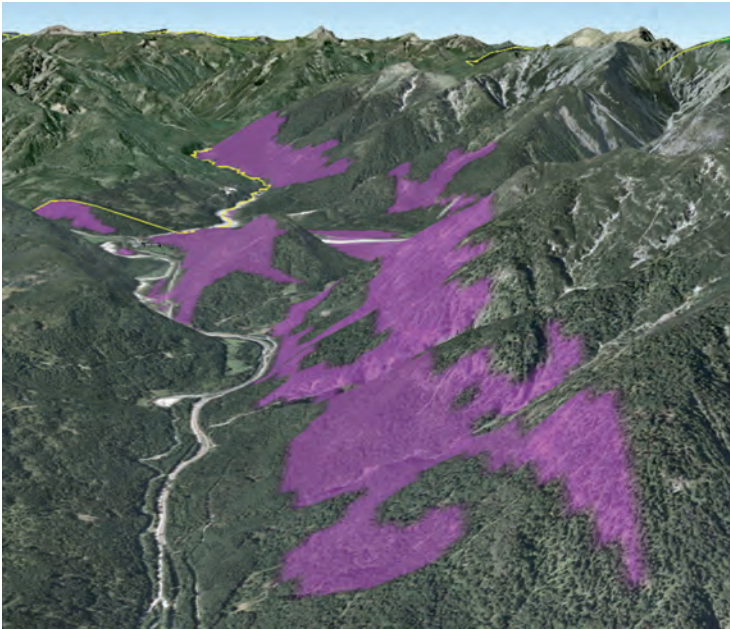
Abb. 19: Xerotherme Kiefernwaldvegetationskomplexe (violett; nicht vollständig) auf Hauptdolomithängen an der Südabdachung des Ammergebirges/Obb. (Blick loisch aufwärts nach Westen; mit Griesen, Ofenberg, Friedergries). Gelbe Linie: Staatsgrenze (Basis: GoogleEarth, Bearbeitung A. Ringler 2015).
