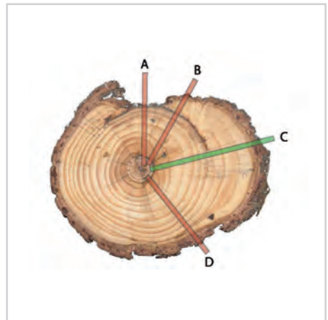
Abb. 23 a. u. b: Pinus uncinata auf dem Murkegel Bärenrufe bei Nenzing/Vorarlberg. Habituell sind diese Bäume von Spirken auf Ammergau und Allgäuer Murkegeln nicht zu unterscheiden. Die Spirkenstammscheibe mit verschiedenen Bohrspänproben zeigt die arttypische Resilienz gegenüber Elementarereignissen und einen deutlichen Jahresringzuwachs nach starker Murgangsverletzung (Fotos: M. Neumann/Stoffel & Bollschweiler aus NEUMANN 2011).
