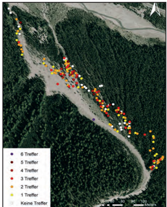
Abb. 37 a u. b: Altersstruktur von Spirken im Murggebiet Val Bruna (Schweizer Nationalpark).
