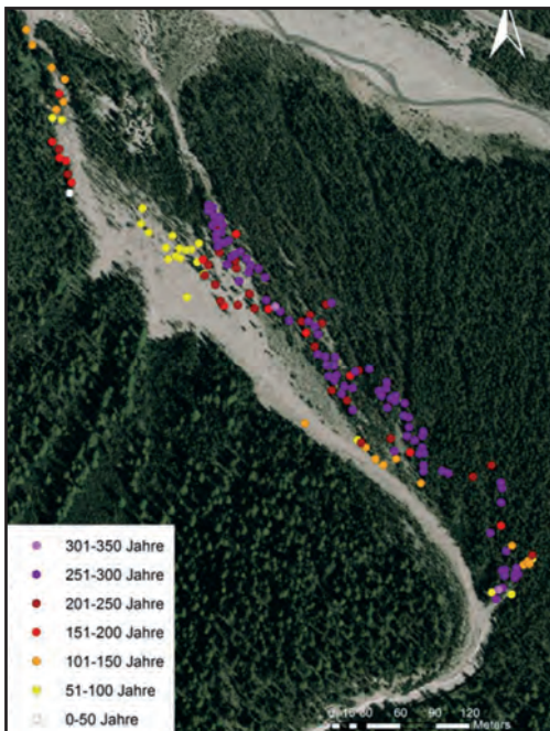
Abb. 37 a u. b: Altersstruktur von Spirken im Murggebiet Val Bruna (Schweizer Nationalpark).
