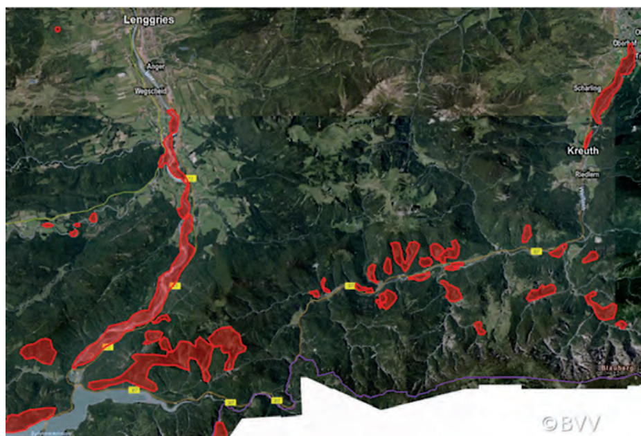
Abb. 14: Karbonatkiefernwald-Biotopkomplexe zwischen Weißbach und Isar/Obb.. (Basis: BVV, Bearbeitung A. Ringler 2015).
