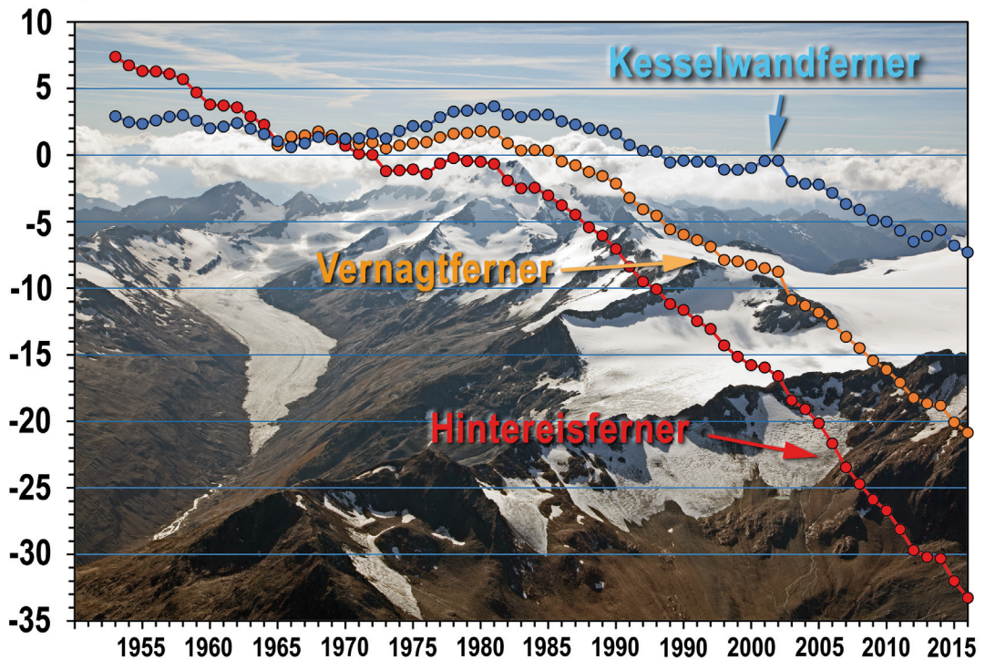
Abb. 3: Kumulative jährliche spezifische Massenbilanzen, bestimmt nach der glaziologischen Methode, für drei Gletscher im hinteren Ötztal. Die Kurven dokumentieren die jährliche mittlere Dickenänderung des Eiskörpers.
