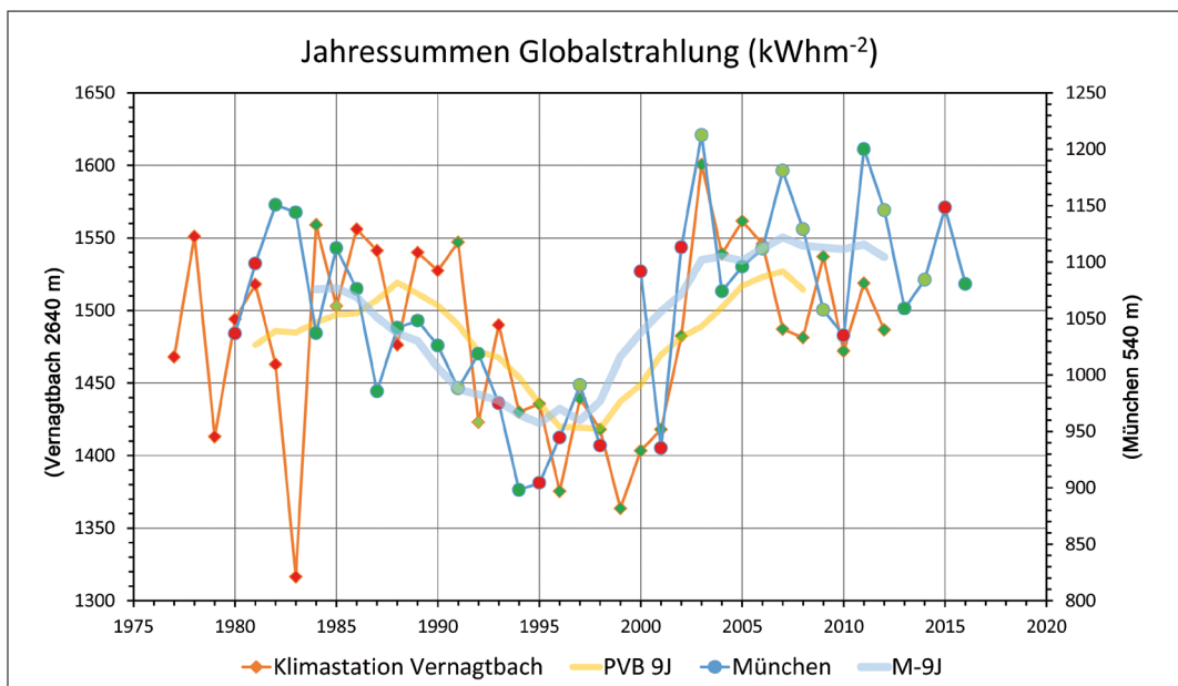
Abb. 8: Jahressummen der solaren Einstrahlung gemessen an der Klimastation Vernagtbach (PVB) und auf dem Dach des Meteorologischen Instituts der Universität München im Zeitraum von 1976 bis 2016 im Vergleich. Grün markierte Messwerte basieren auf vollständigen Messreihen und haben eine geringe Fehlerquote, bei mit rot markierten Werten weisen die Messdaten Lücken auf, die durch Schätzwerte ergänzt wurden. Daher besitzen sie einen Fehlerbalken von mehr als 100 \text{ kWhm}^{-2} .
