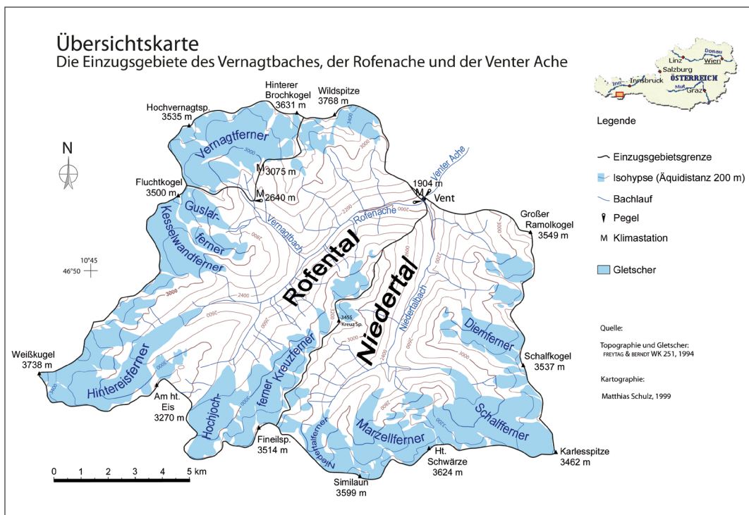
Abb. 15: Schematische Karte des Einzugsgebiets der Venter Ache am Pegel Vent mit einigen seiner Teileinzugsgebiete und den darin befindlichen Gletscherflächen, gelegen im hinteren Ötztal in Österreich. Oben das Einzugsgebiet der Pegelstation Vernagtbach auf 2635 m mit einer Fläche von 11,4 km 2 . Der Vernagtbach mündet in die Rofenache, deren Abfluss bei einer Gesamtfläche des Einzugsgebietes von 98 km 2 am Pegel Rofenache in Vent gemessen wird. Die blauen Flächen zeigen die Ausdehnung der Gletscher im Jahre 1994. (Aus BRAUN & ESCHER-VETTER 2013)
