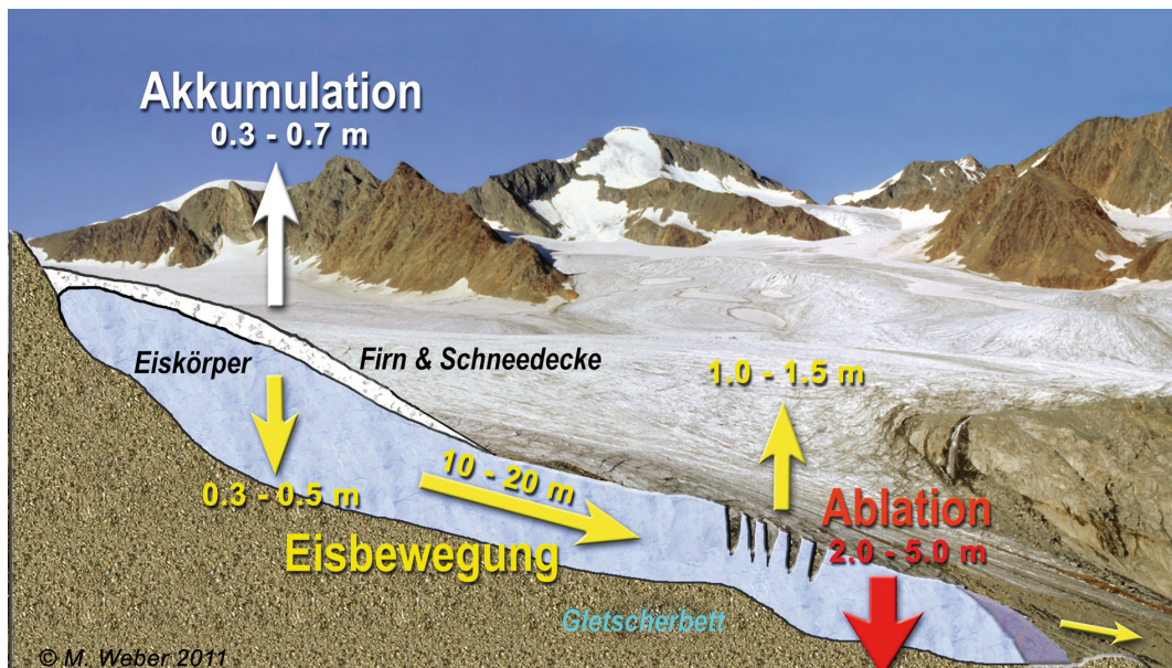
Abb. 5: Veränderung der Form des Eiskörpers durch das Zusammenwirken der Prozesse Akkumulation (Massenzuwachs), Ablation (Massenverlust durch Schmelze) und die Umverteilung von Masse durch die Eisbewegung. Die Zahlenangaben entsprechen den Beobachtungen am Vernagtferner in den 1980er und 1990er Jahren.
