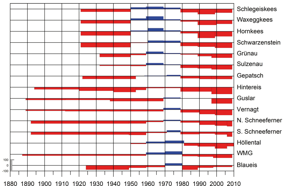
Abb. 2: Veränderung ausgewählter Ostalpengletscher seit dem Ende des 19. Jahrhunderts basierend auf photogrammetrisch erhobenen Volumendifferenzen. Dargestellt sind die jährlichen Veränderungen der mittleren Höhe der Gletscheroberfläche [cm pro Jahr, rot: negativ, blau: positiv] der Basis der geodätischen Bestimmung des Massenhaushaltes der Gletscher nach FINSTERWALDER & RENTSCH (1981), ESCHER-VETTER (2005), aktualisiert durch C. MAYER.
