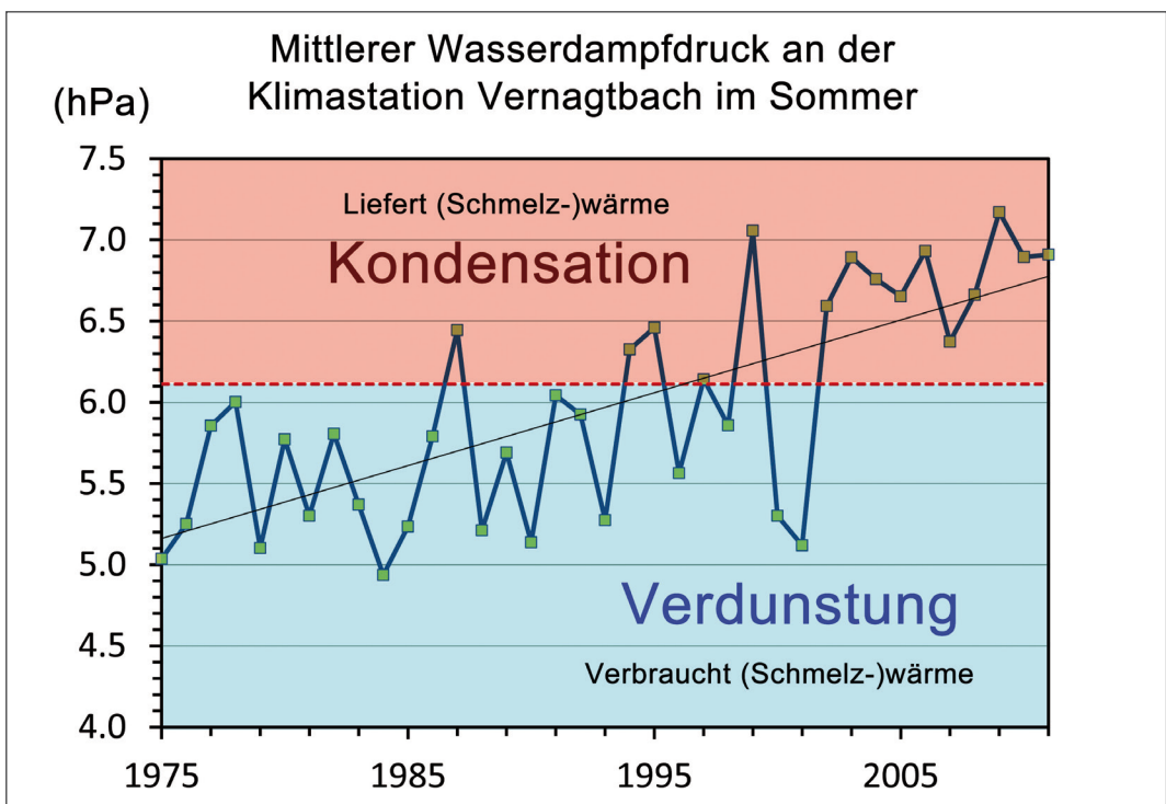
Abb. 11: Mittlerer Wasserdampfdruck an der Klimastation Vernagtbach im Sommer. Der Sättigungsdampfdruck an der schmelzenden Schnee- und Eisoberfläche beträgt 6.1 hPa. Liegt der Wasserdampfdruck darunter (bis Ende der 1990er Jahre), herrschen Verdunstungsbedingungen vor mit einer Reduktion der Schmelzwärme. Liegt der Wasserdampfdruck über diesem Schwellenwert, wird zusätzliche Schmelzwärme durch Kondensation freigesetzt.
