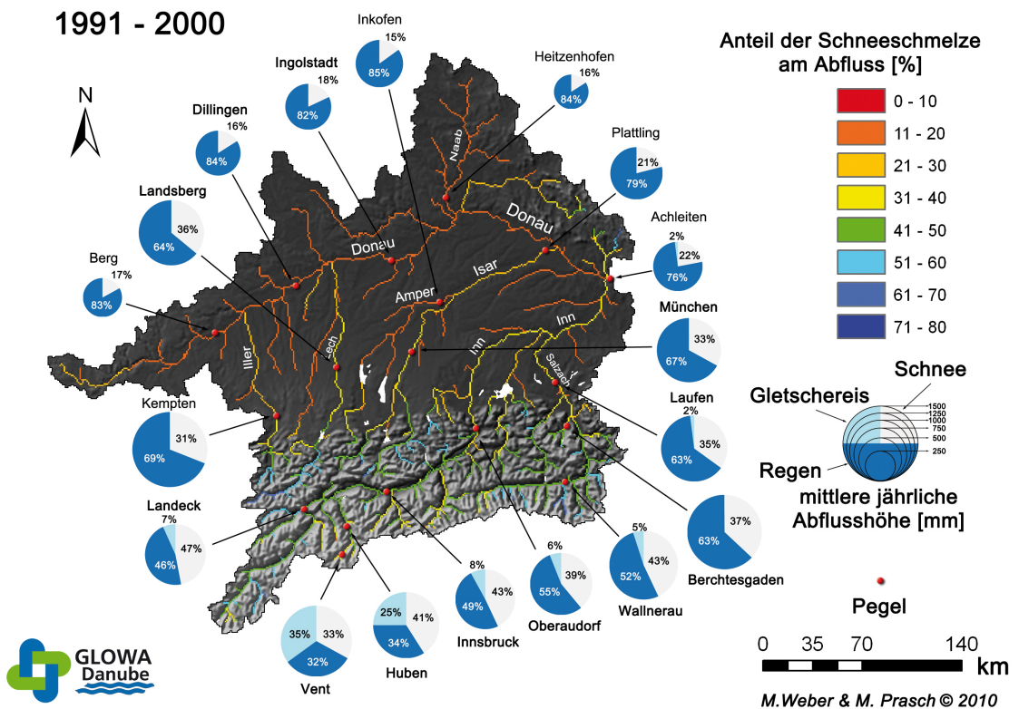
Abb. 18: Mittlere jährliche Anteile der Schneeschmelze in den Flüssen im Einzugsgebiet der Donau, definiert durch den Pegel Passau-Achleiten für die Dekade 1991-2000. Zusätzlich werden an ausgewählten Pegelstellen die jährlichen spezifischen Abflusshöhen sowie ihre Quellanteile nach Regen, Schnee- und Gletscherschmelze in Form von Kuchendiagrammen angegeben. Es handelt sich um Resultate einer hydrologischen Modellrechnung auf der Basis von Beobachtungsdaten.
