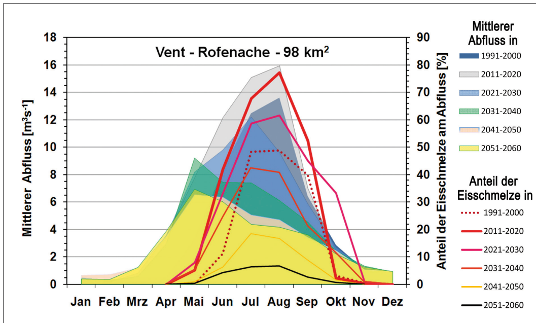
Abb. 17: Mittlere Abflüsse und Anteile der Eisschmelze am Pegel Rofenache / Vent in den Dekaden 1991-2000 bis 2051-2060.
