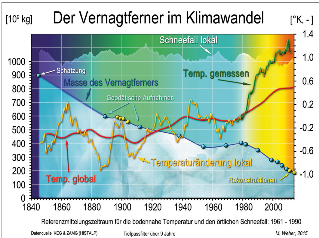
Abb. 4: Der Vernagtferner im Klimawandel 1845 bis 2016. Die aus den geodätisch bestimmten Volumendifferenzen berechneten Massenänderungen (linke Achse, mio Tonnen) sind im Vergleich zu den Abweichungen vom Mittelwert 1961 – 1990 der globalen Mitteltemperatur (rot), der lokal für die Pegelstation Vernagtbach (2640 m ü. NN) nach BÖHM & HIEBL (2013) rekonstruierten (gelb), und der seit 1974 gemessenen (grün) bodennahen Lufttemperatur dargestellt (alle bezogen auf die rechte Achse in Kelvin). Im Hintergrund ist zusätzlich das dimensionslose Verhältnis des lokalen Schneeeintrags in Relation zu dem im Referenzzeitraum 1961-1990 angegeben (rechte Achse). Auf sämtliche meteorologische Messreihen wurde ein Tiefpassfilter von 9 Jahren angewendet, um die Antwortzeiten des Gletschers zu simulieren.
