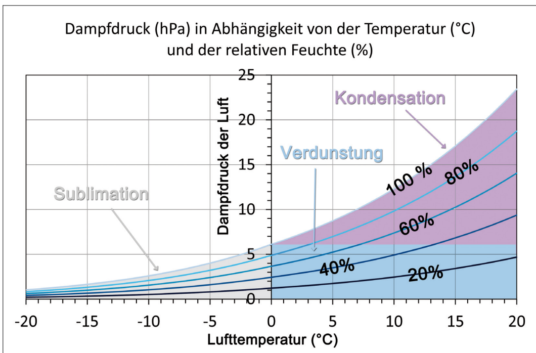
Abb. 10: Dampfdruck der Luft in Abhängigkeit von der Lufttemperatur und der relativen Feuchte. Die Sättigung der Luft an Wasserdampf ist bei 100% relativer Luftfeuchtigkeit erreicht. Über einer schmelzenden Gletscherfläche mit einer Oberflächentemperatur von maximal 0°C kann in dem blau markierten Bereich bei einem ausreichend hohen Energieangebot Wasser auf dem Eis verdunstet werden. Im roten Bereich dagegen kondensiert Wasserdampf an der kalten Oberfläche, dabei wird die zuvor für das Verdunsten verbrauchte Energie wieder freigesetzt. Im grau markierten Bereich ist allein Sublimation (der direkte Übergang von der festen in die dampfförmige Phase) möglich, dabei wird jedoch das Achtfache an Energie wie zum Verdunsten verbraucht. Dank der höheren Temperaturen im Klimawandel kommt es auch in nicht gesättigter Luft zur Kondensation.
